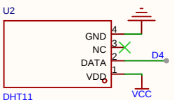
DHT11
