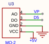
MQ-2
