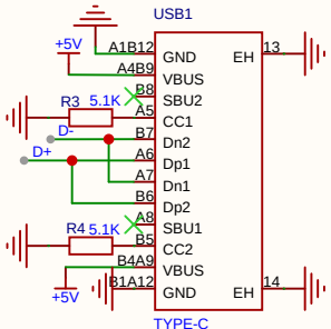
TYPE-C 下载电路
