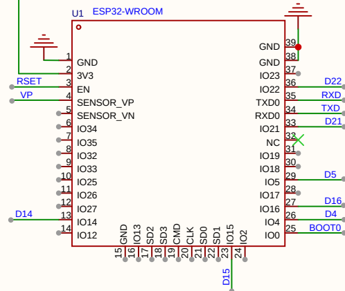
ESP32主控板
