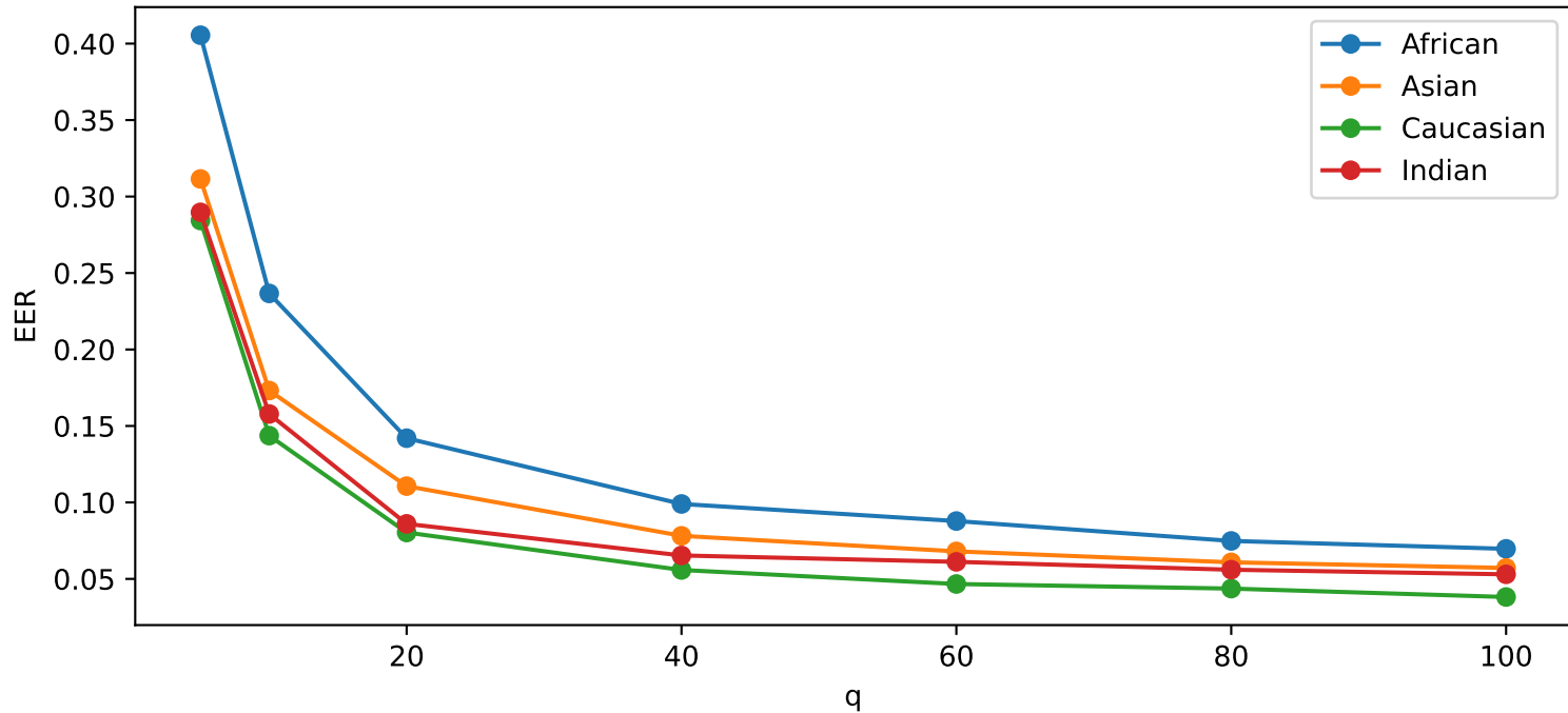
EER — JPEG Compression
