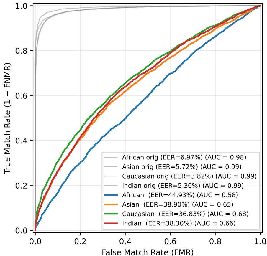
ROC — Motion Blur (k=29)
