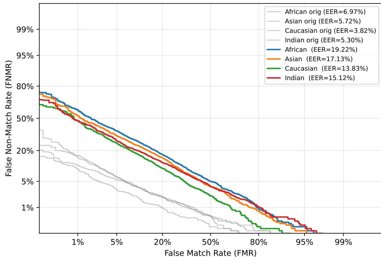
DET — Motion Blur (k=9)
