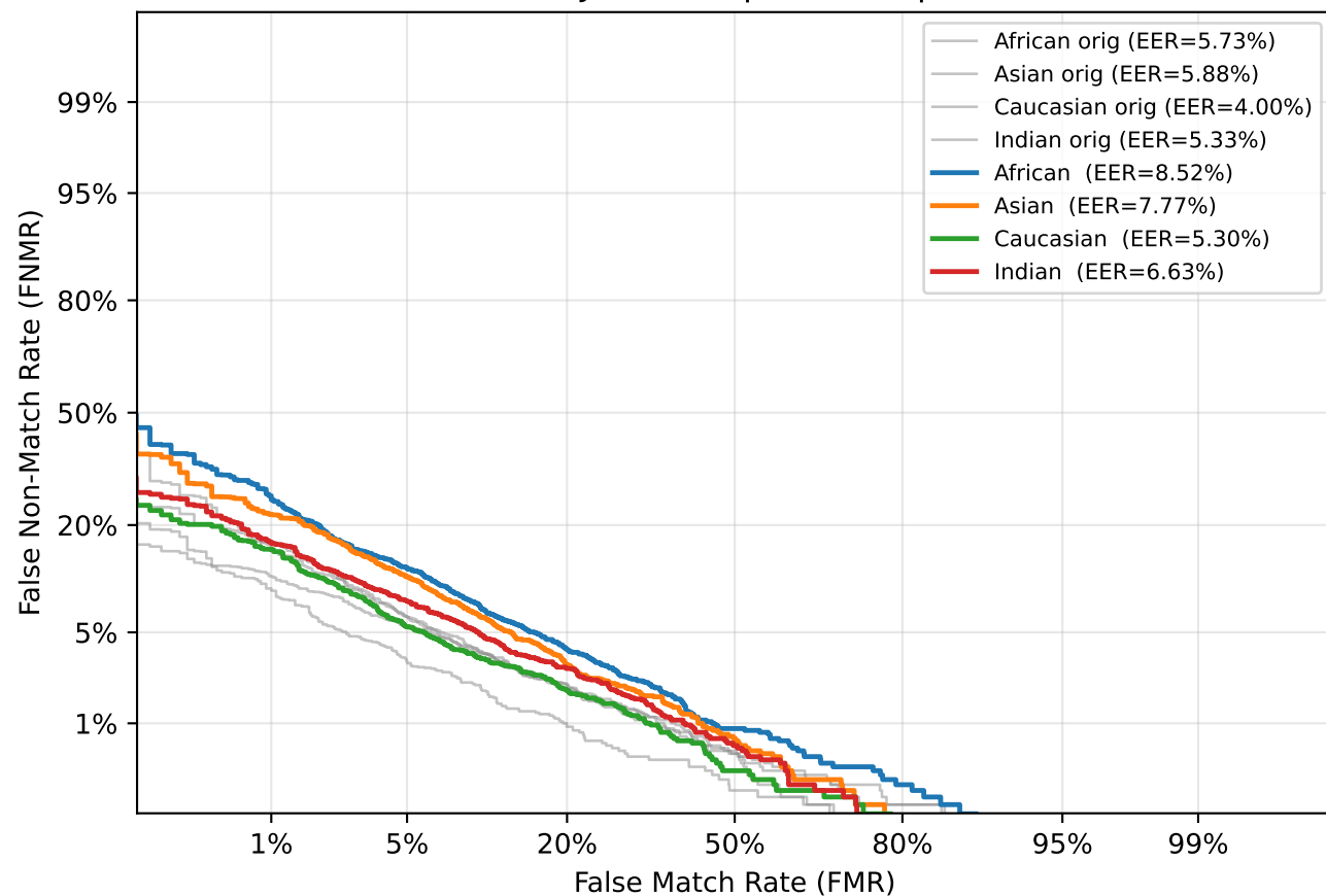
DET — JPEG Compression (q=40)
