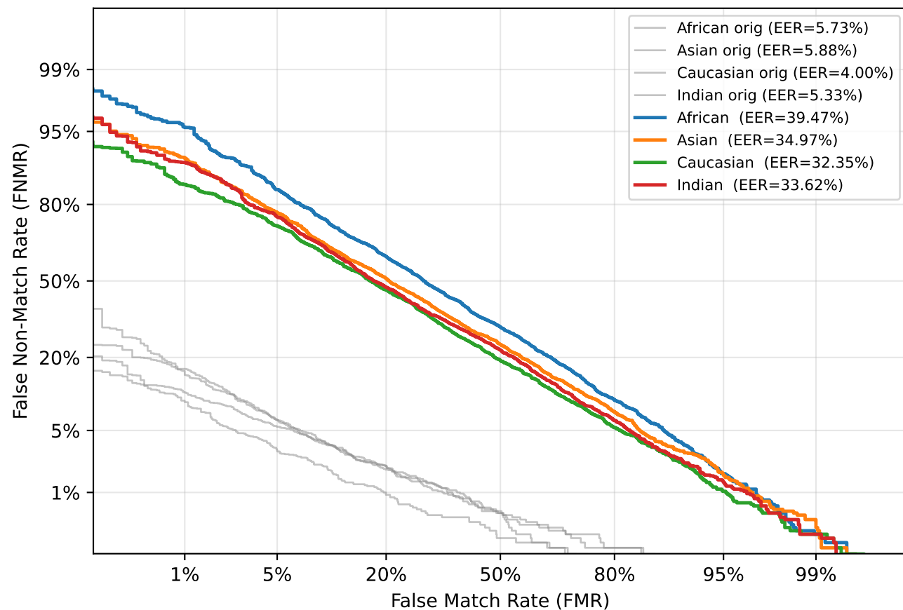
DET — Motion Blur (k=21)
