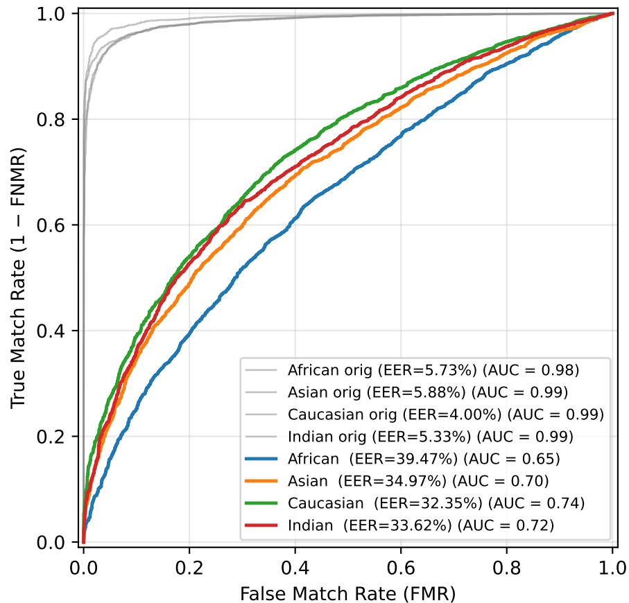
ROC — Motion Blur (k=21)
