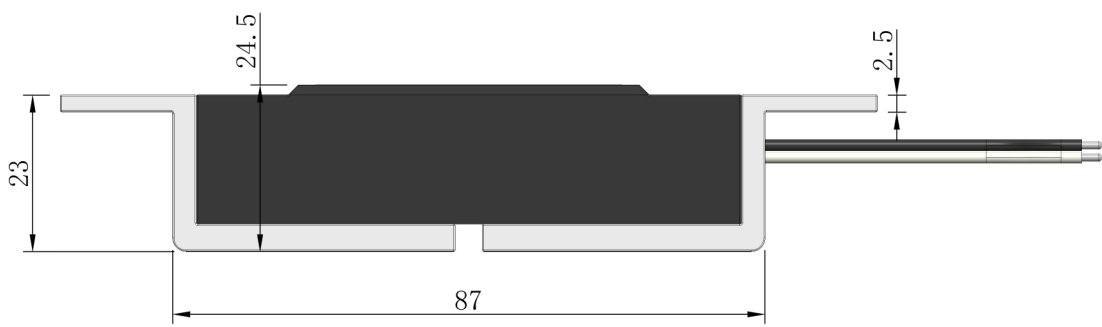
电磁铁 侧面
