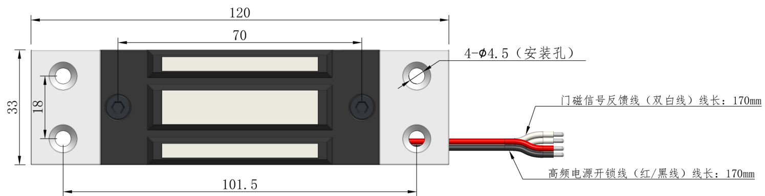
电磁铁 正面
