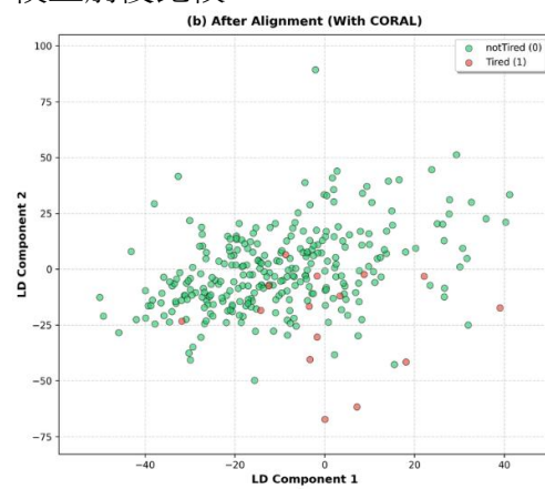
圖 42. B 同學 LDA 結果圖
