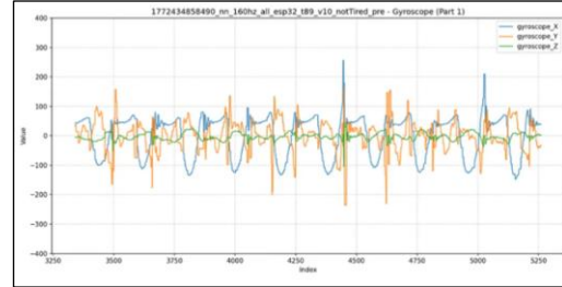
圖 10. 原始波形(陀螺儀)
