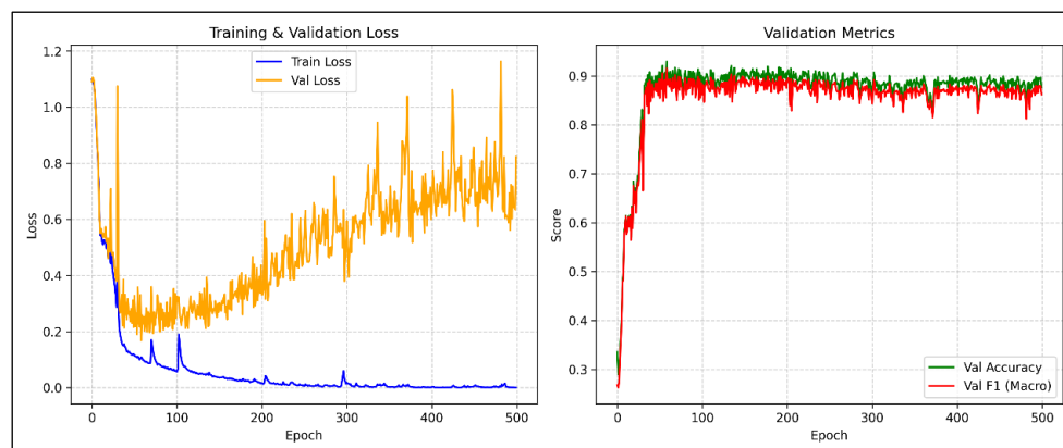
圖 38. 模型訓練與驗證損失及驗證集評估指標
