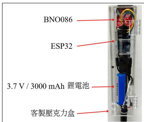
圖 4. 登山杖嵌入式感測模組原型
