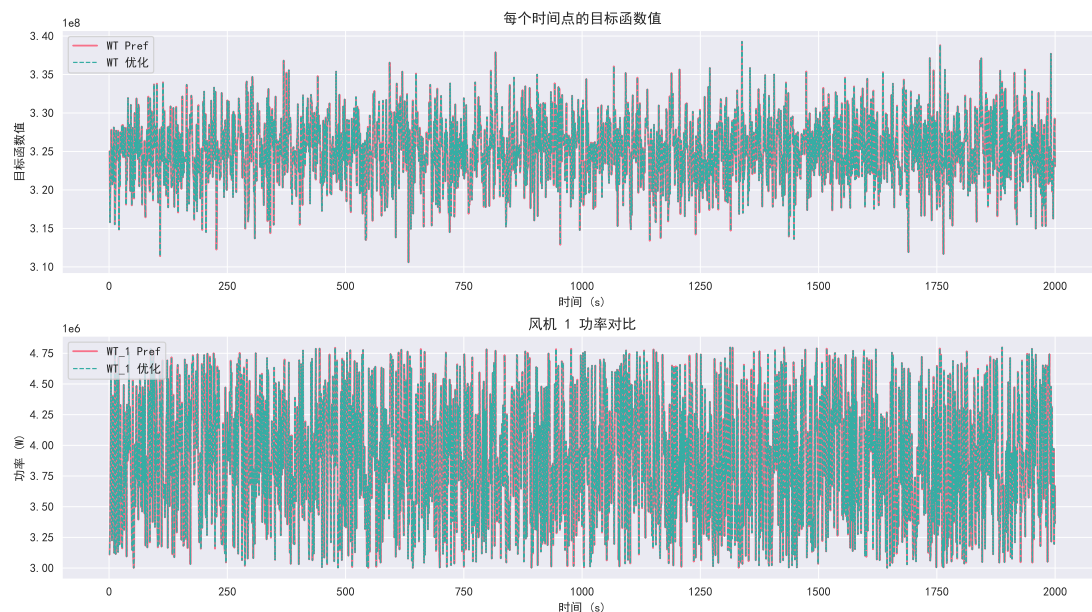
图 4-5 优化调度功率对比
