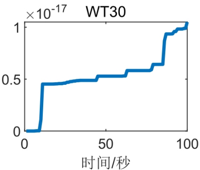
塔架累计疲劳损伤程度
