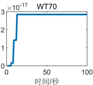
塔架累计疲劳损伤程度
