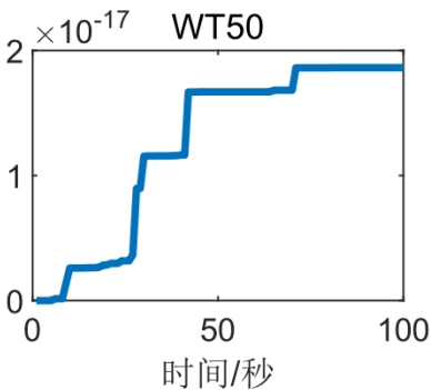
塔架累计疲劳损伤程度
