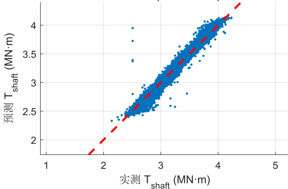
主轴扭矩 ( R^2 = 0.9691 )
