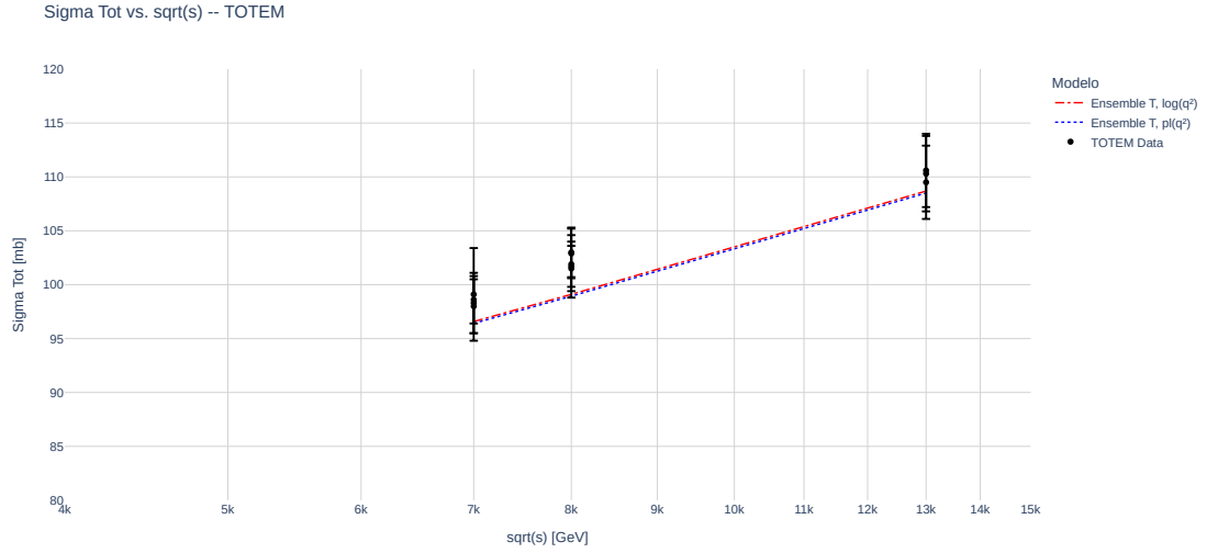
Figure 4: Resultados eiconalizados com fit global para \sqrt{s}=7, 8 e 13 TeV para o ensemble TOTEM
