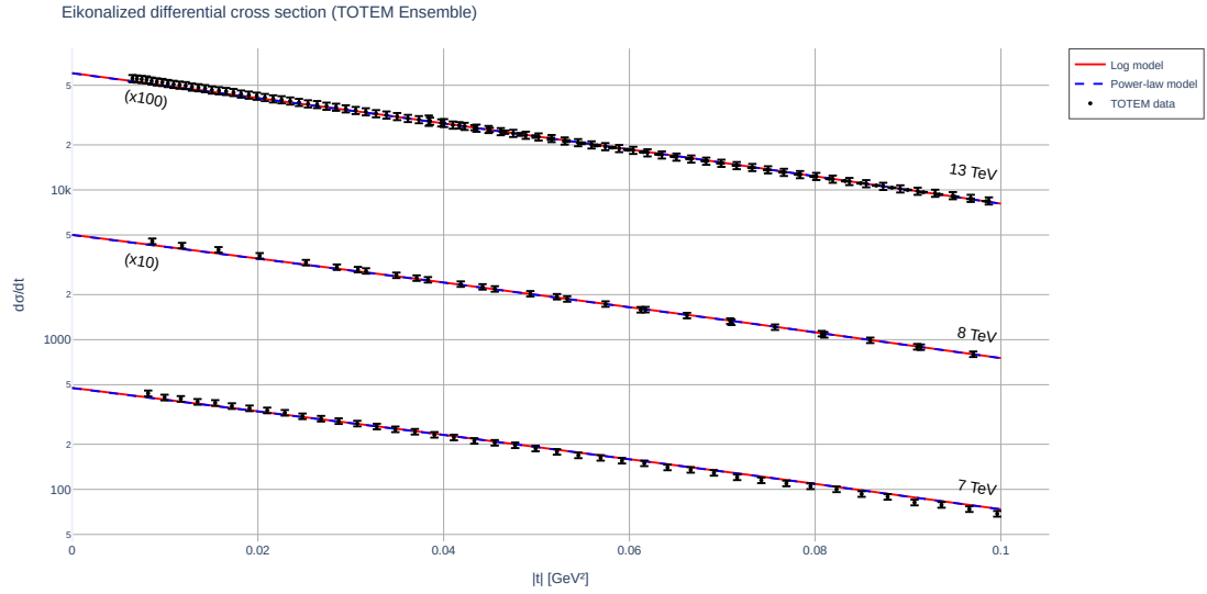
Figure 2: Resultados eiconalizados com fit global até q^2 = 0.1 para o ensemble TOTEM
