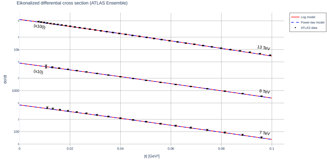
Figure 1: Resultados eiconalizados com fit global até q^2 = 0.1 para o ensemble ATLAS
