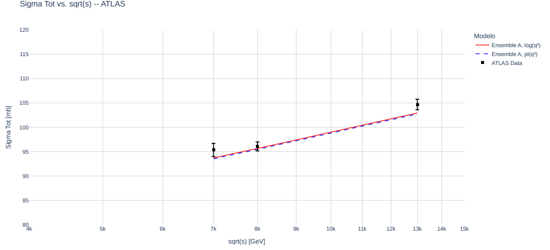
Figure 3: Resultados eiconalizados com fit global para \sqrt{s}=7, 8 e 13 TeV para o ensemble ATLAS
