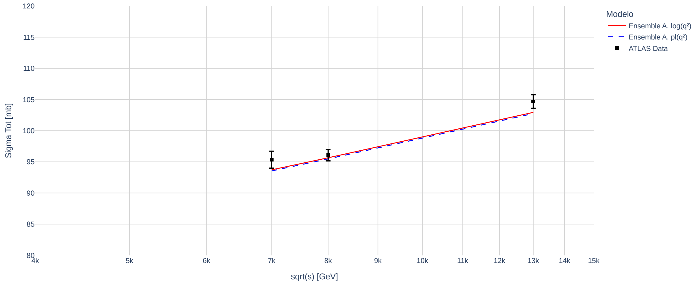
Sigma Tot vs. sqrt(s) -- ATLAS
