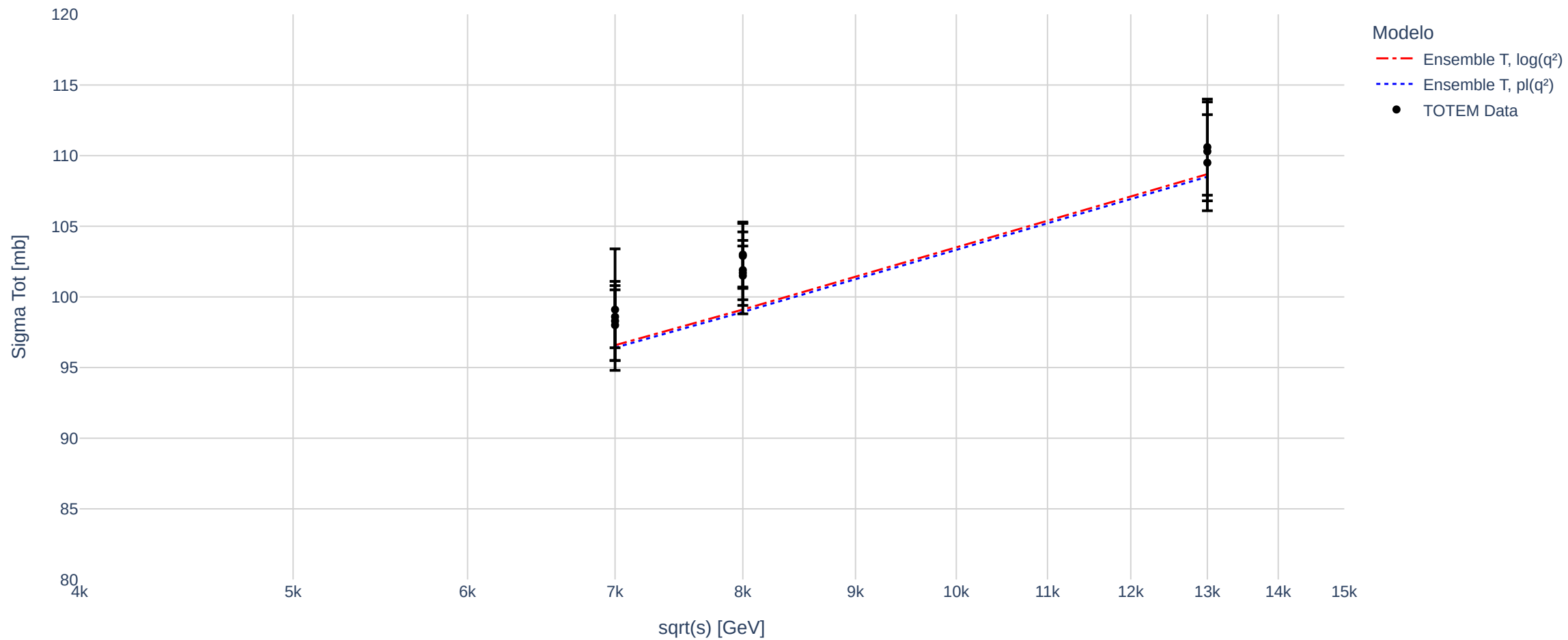
Sigma Tot vs. sqrt(s) -- TOTEM
