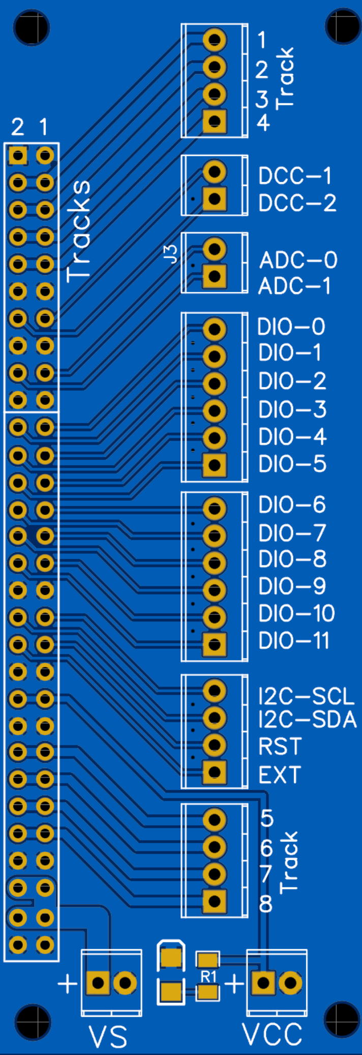
LcsNodes-Extension-Adapter-Socket-B.02.10
