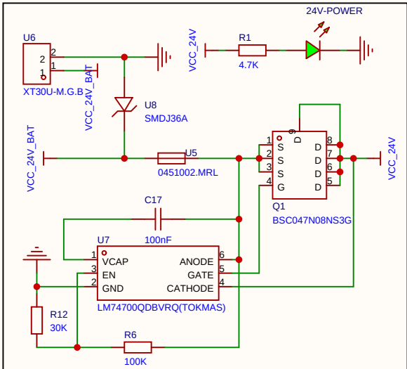
电源输入保护
