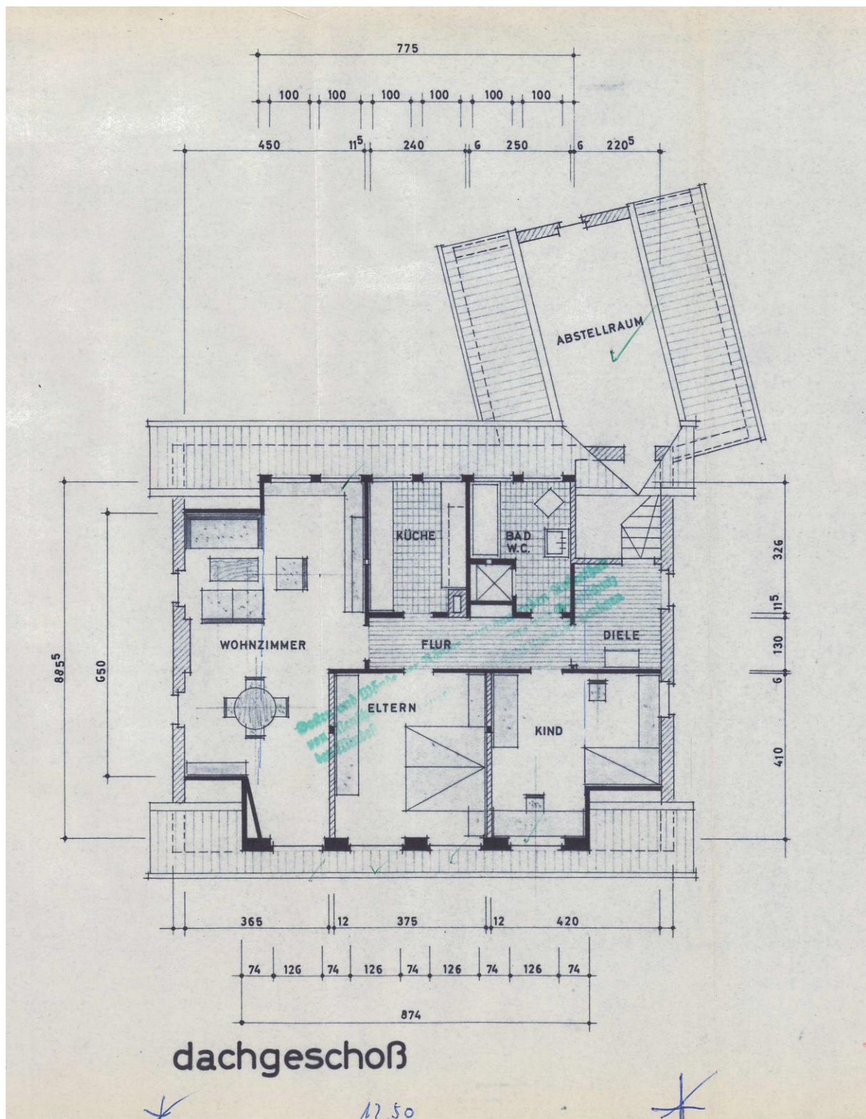
Gebäude 1 (Ausbau des Dachgeschosses im Jahr 1969)
