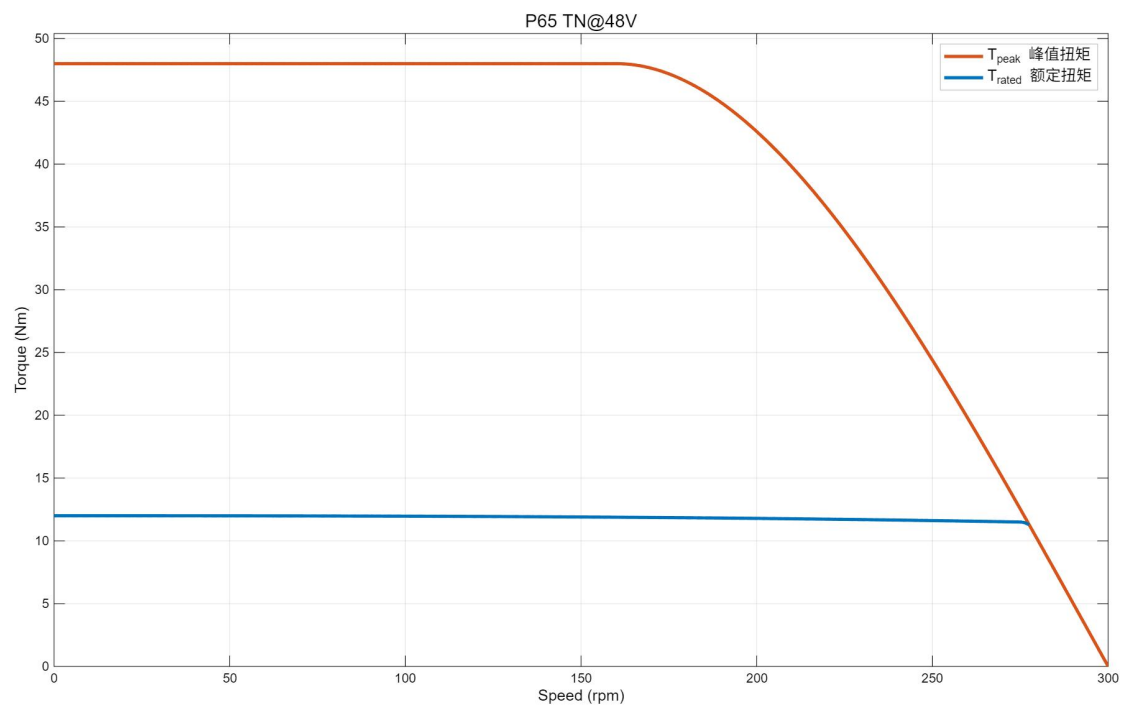
P65 T-n 曲线
