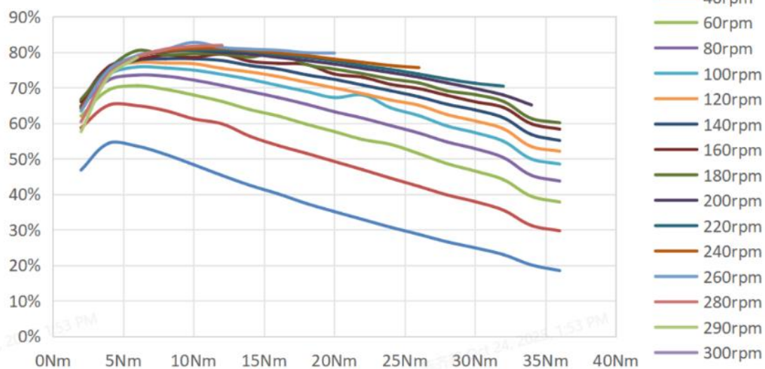
P65 效率曲线
