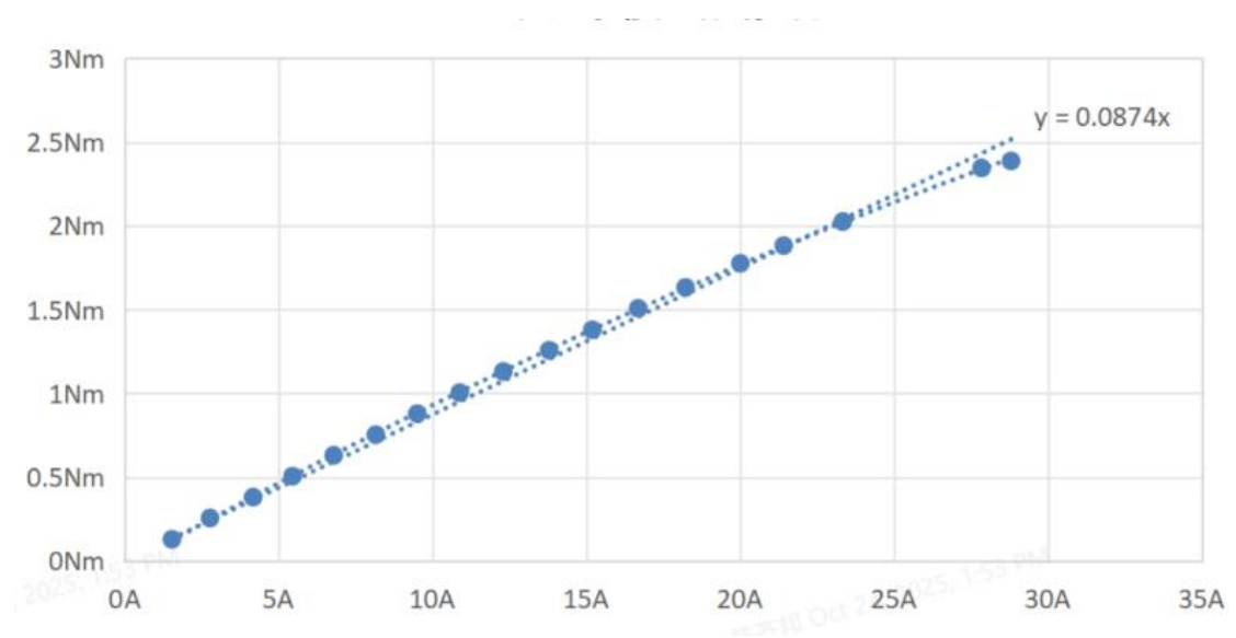
P65 T-i 曲线
