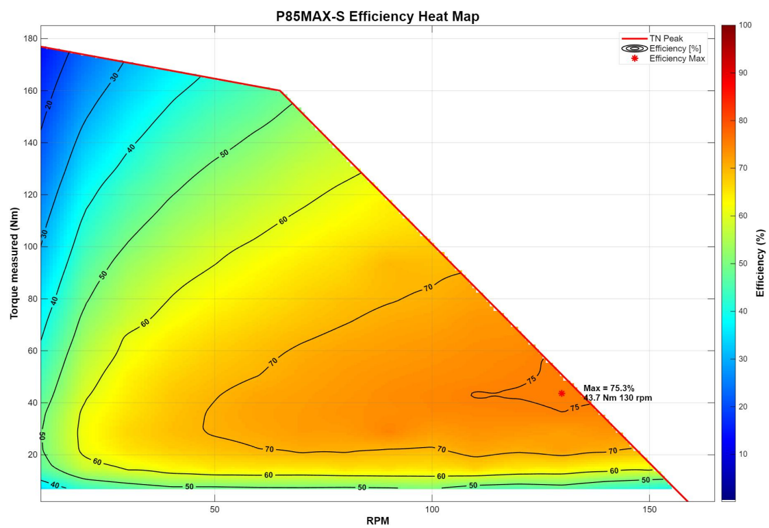
P85MAX-S 效率 map 图
