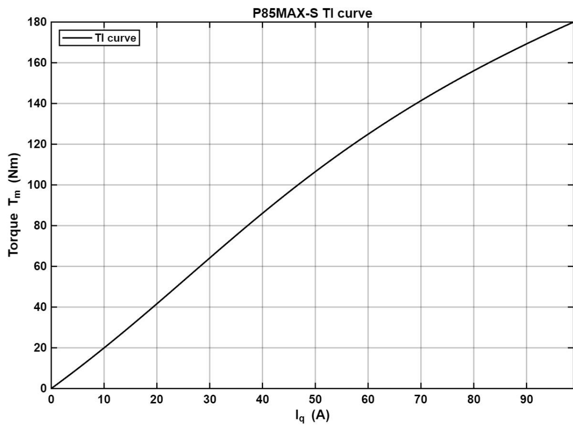
P85MAX-S T-i 曲线
