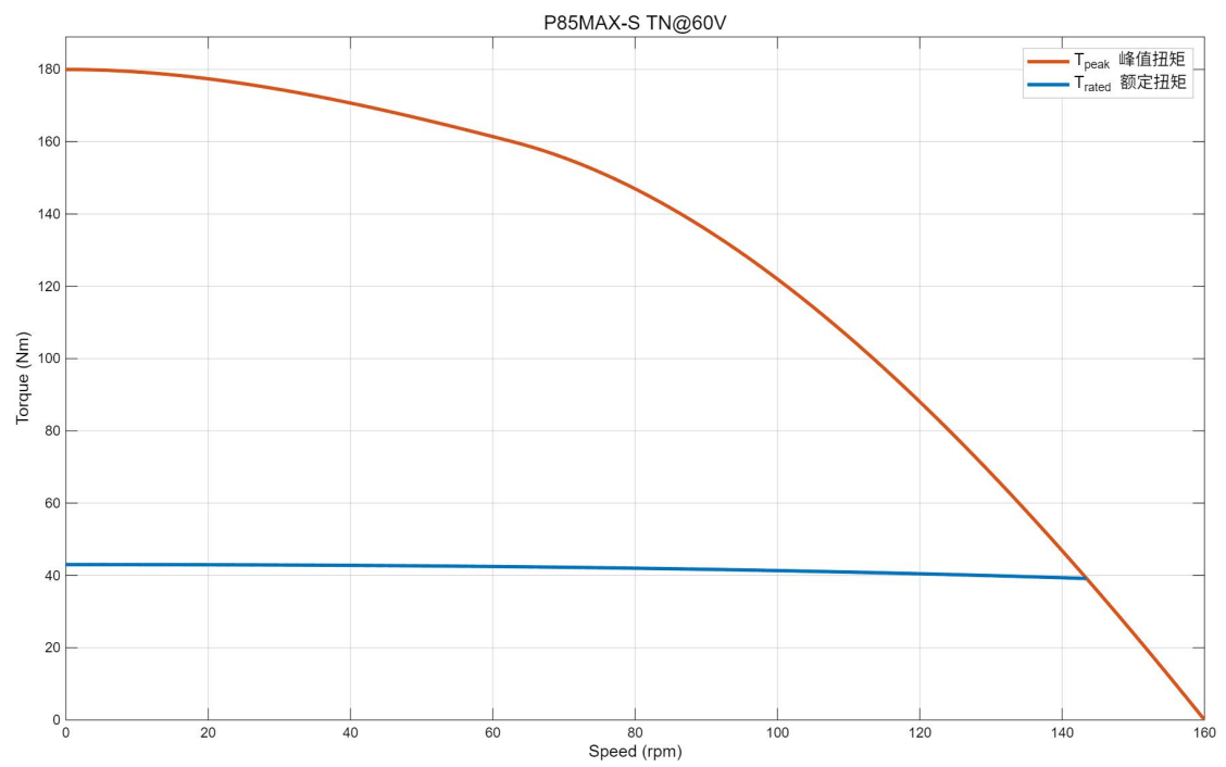
P85MAX-S T-n 曲线
