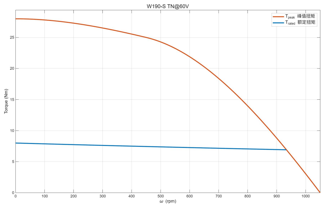
W190-S T-n 曲线
