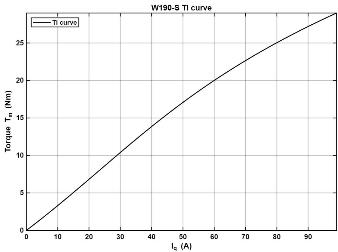
W190-S T-i 曲线
