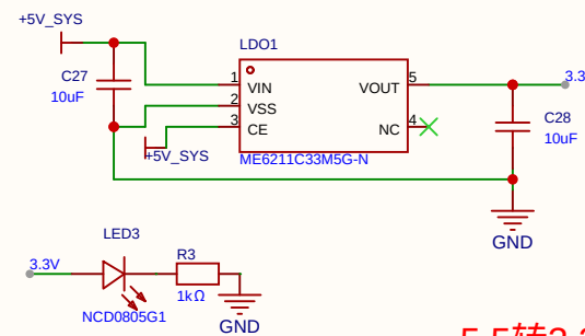
5.5转3.3稳压电路
