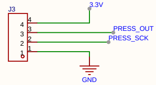
压力检测
