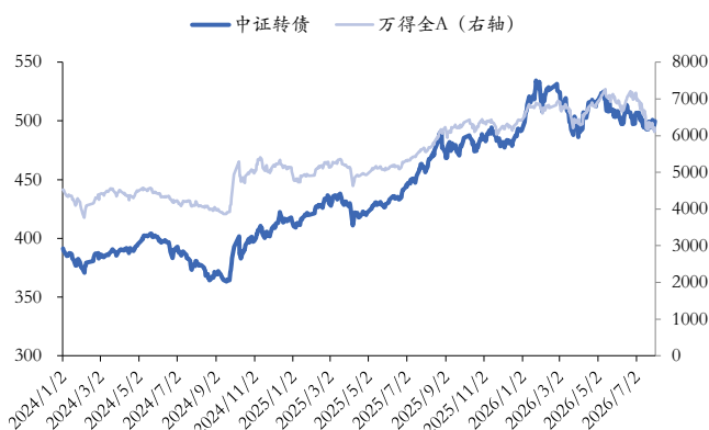
图24: 转债与权益市场表现
