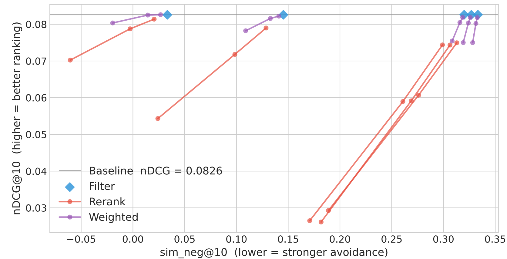
MovieLens 20M
