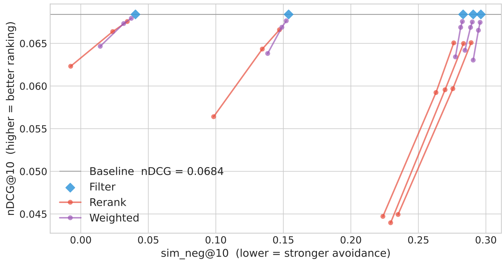
MovieLens 10M
