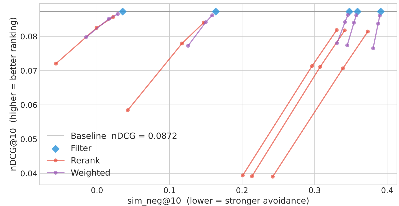
MovieLens 20M
