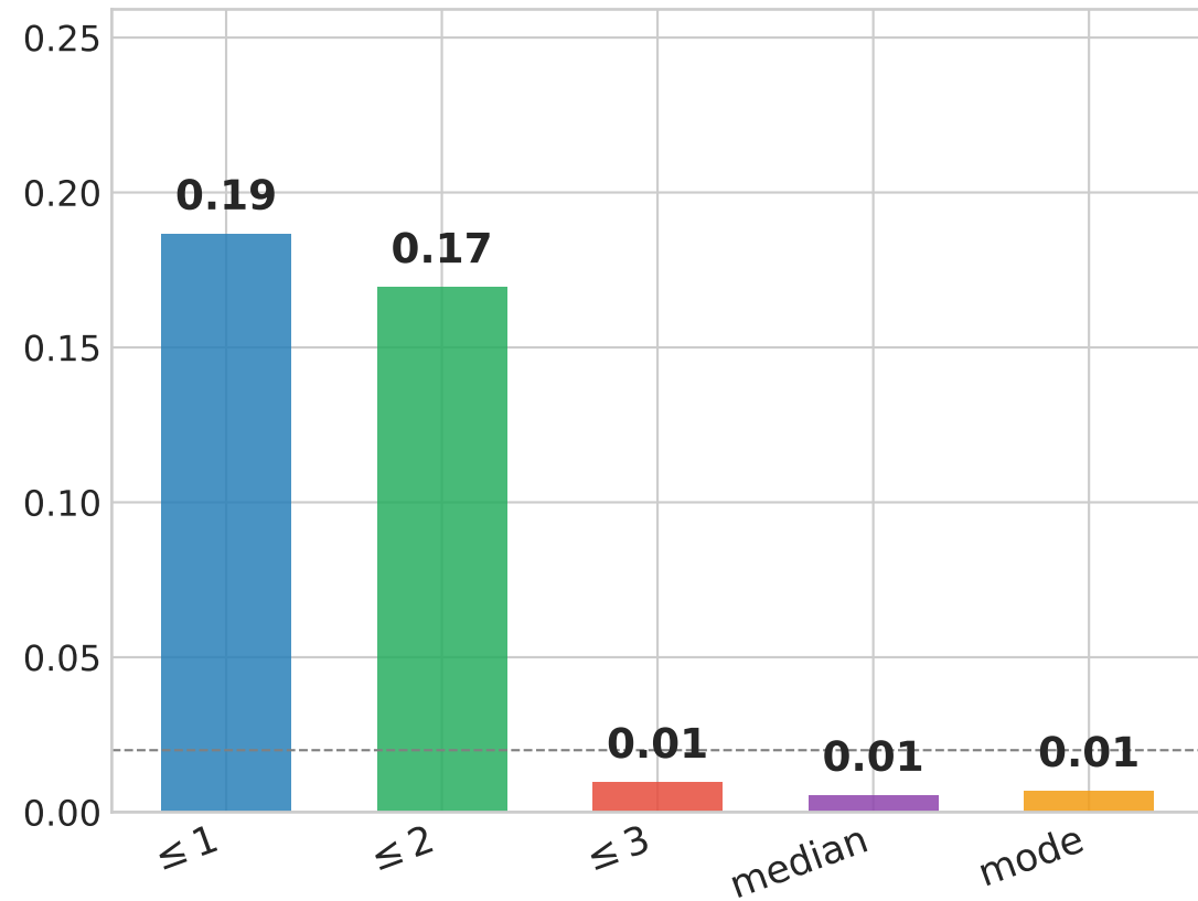
MovieLens 10M
