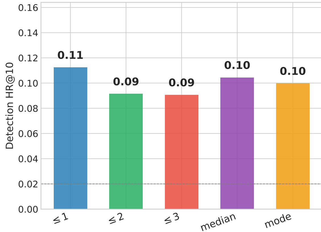
MovieLens 1M
