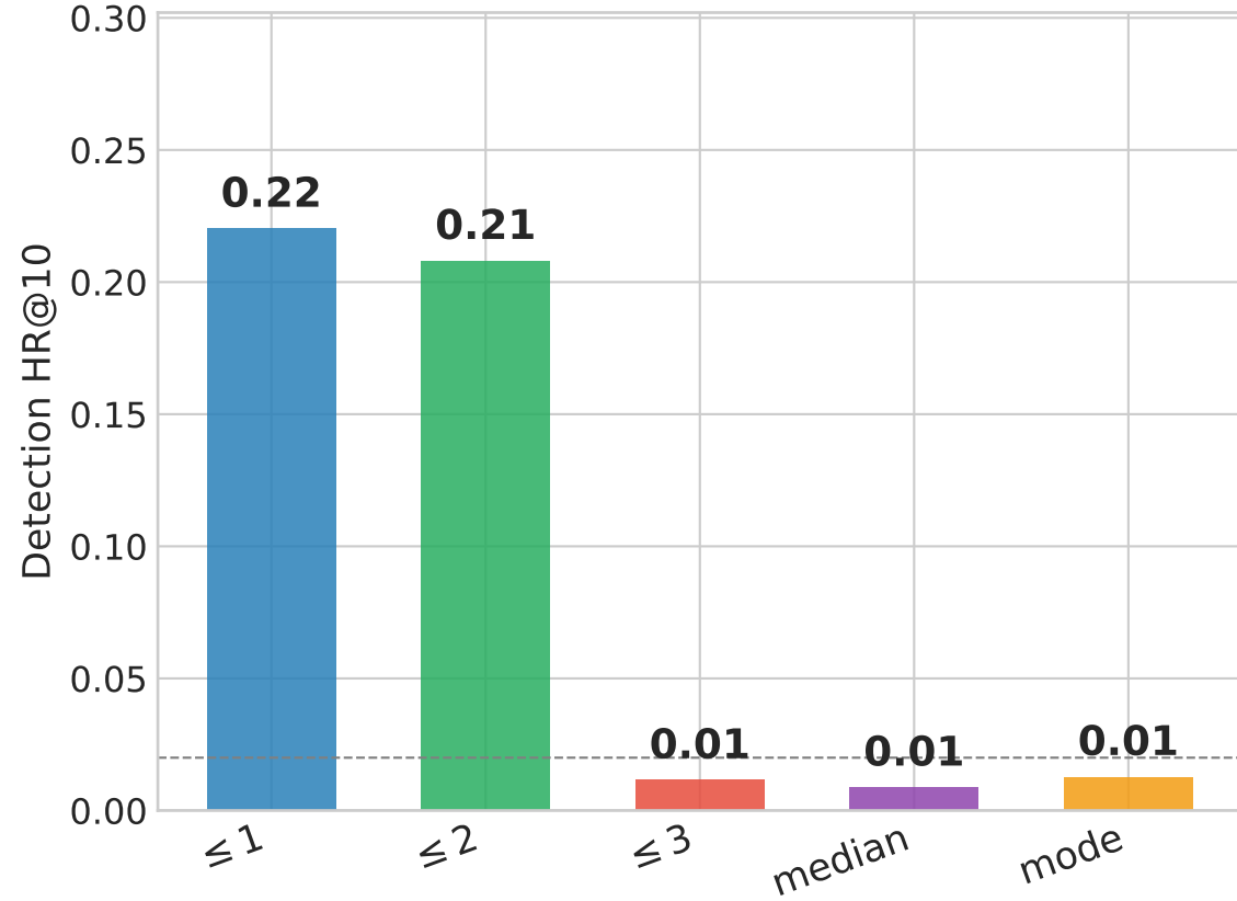
MovieLens 20M
