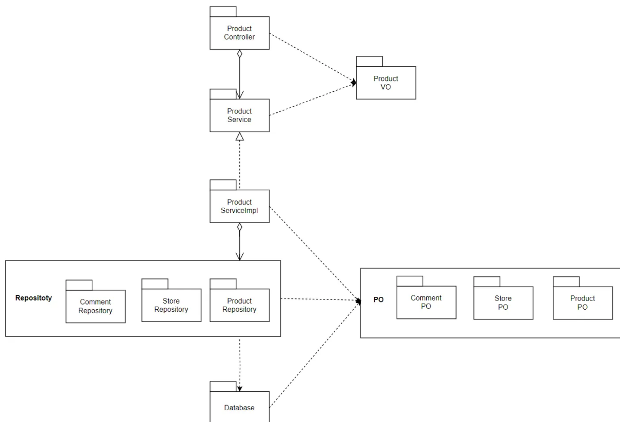
图5.3.2.3 Productbl模块关键类图
