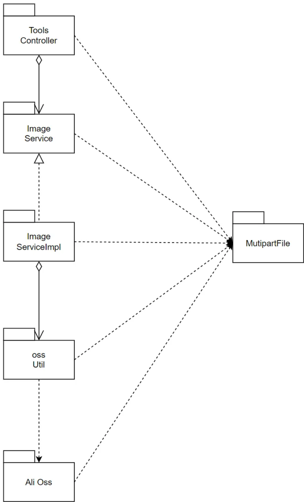
图5.3.2.1 Toolsbl模块关键类图
