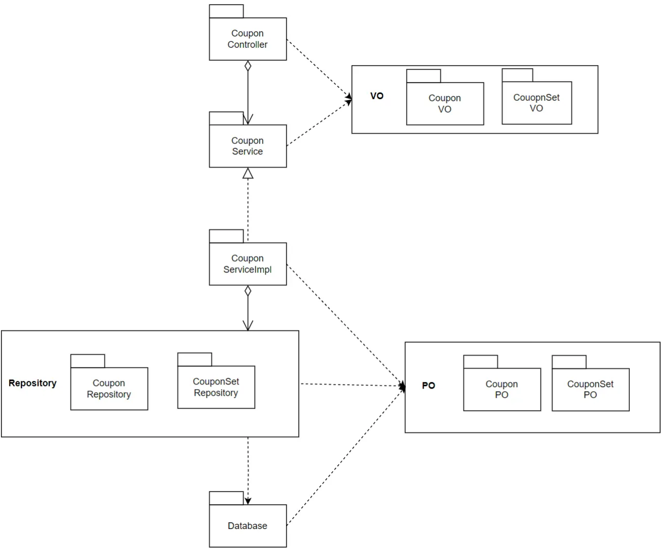
图5.3.2.6 Couponbl模块关键类图
