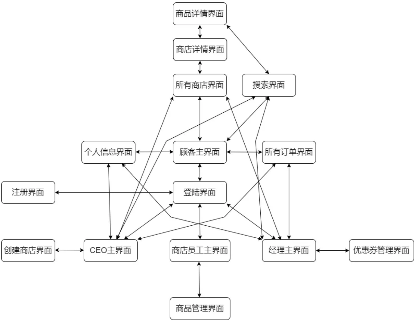
图5.2 用户界面跳转
