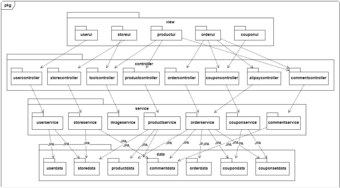
图 3.2 软件体系结构逻辑设计方案
