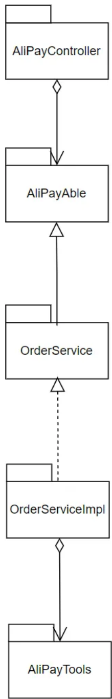
图5.3.2.7 AliPay模块关键类图
