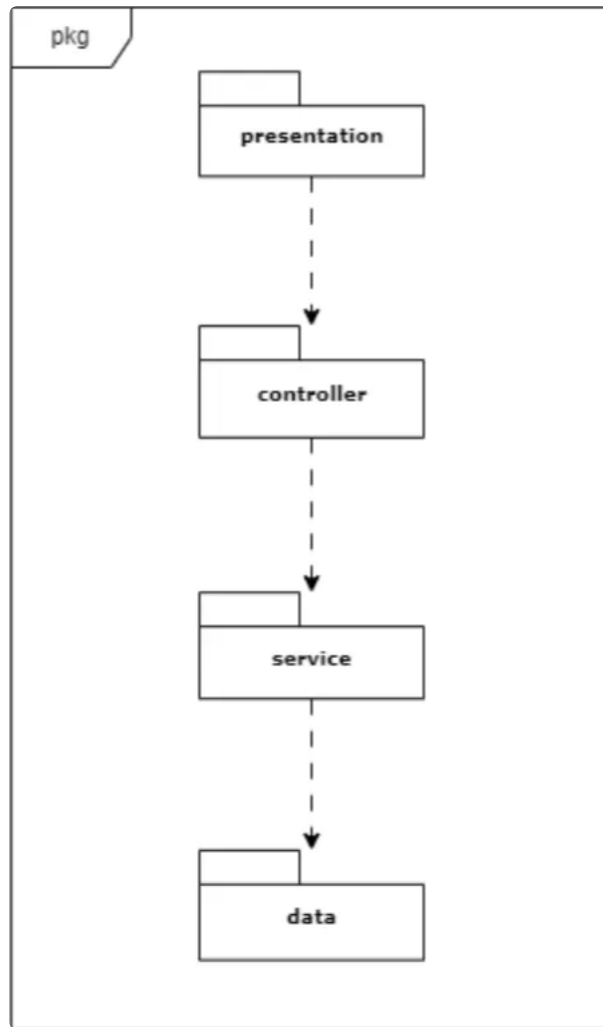
图 3.1 参照体系结构风格的包图表达逻辑视角
