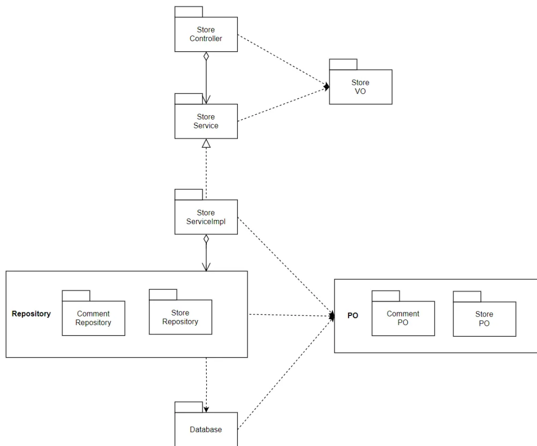
图5.3.2.4 Storebl模块关键类图
