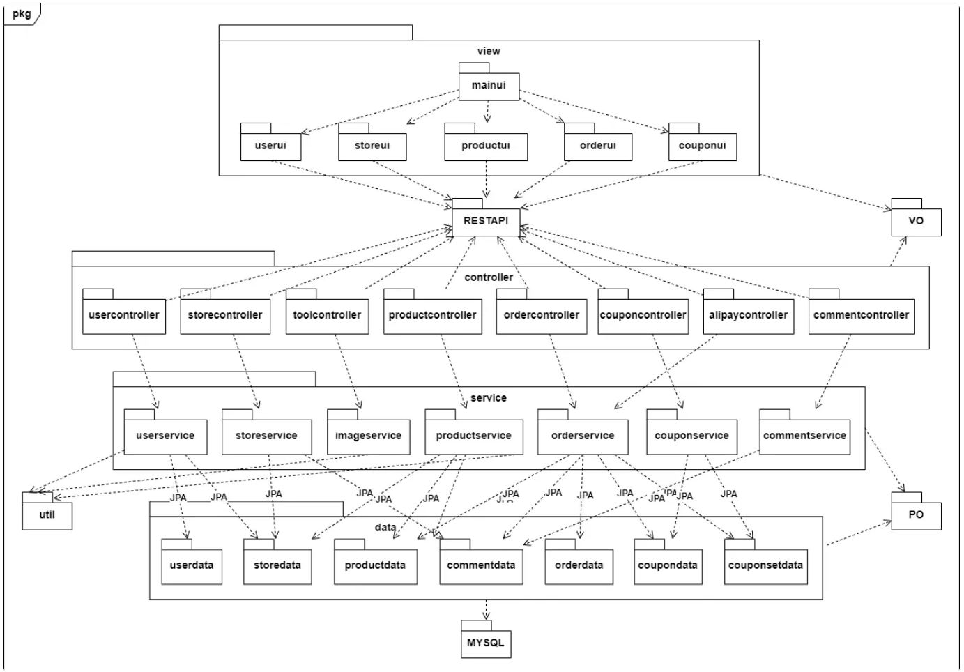
图 4.1 BlueWhale系统开发包图
