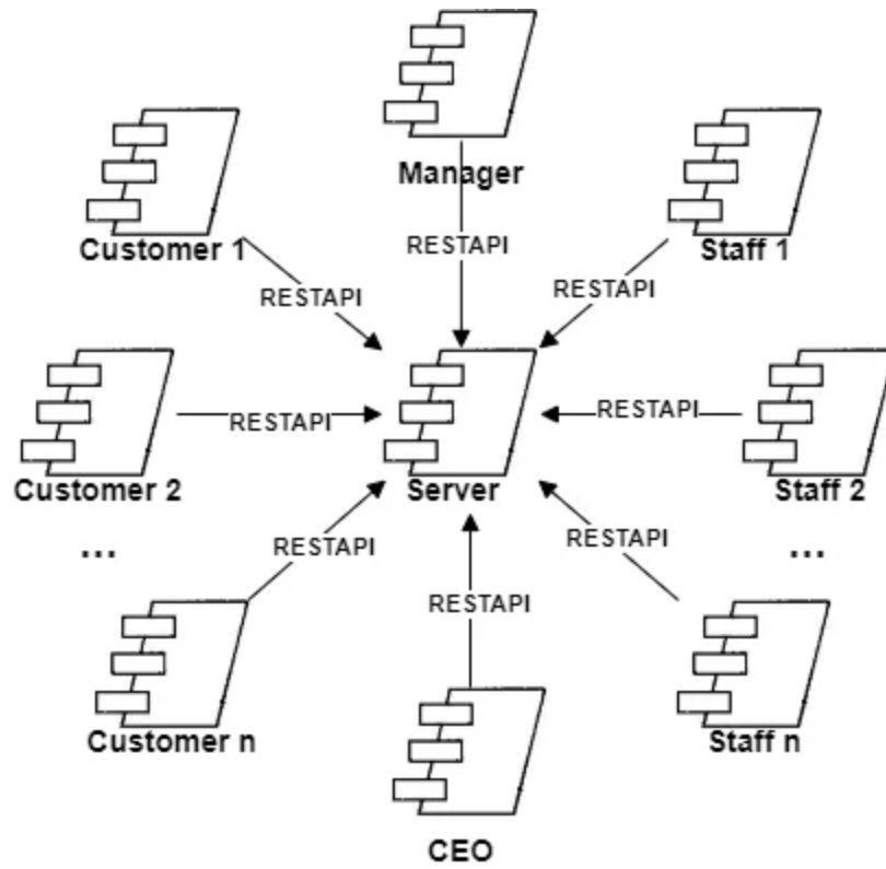
图 4.2.1 进程图
