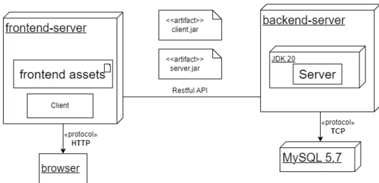
图4.3 部署图
