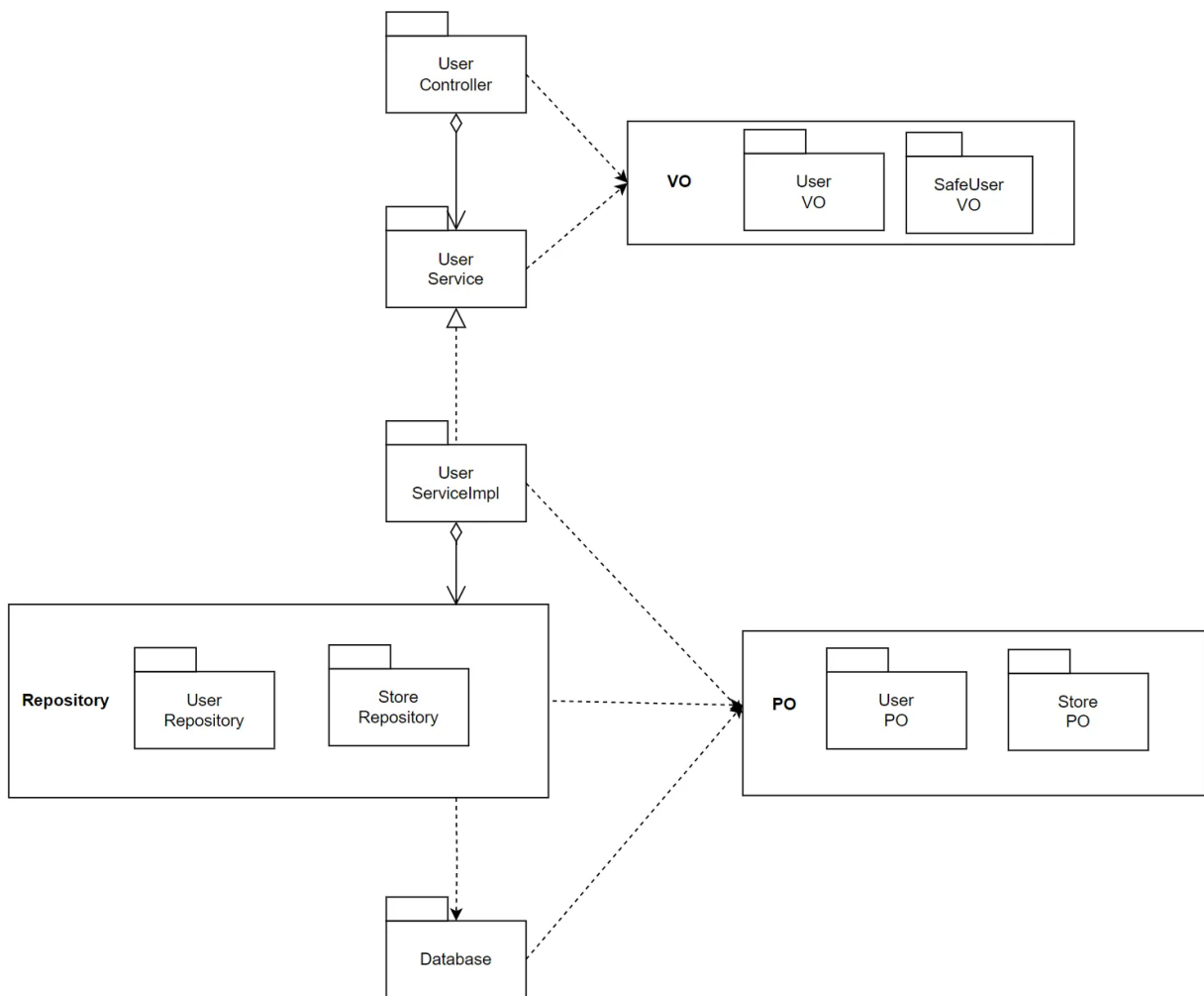
图5.3.2.5 Userbl模块关键类图
