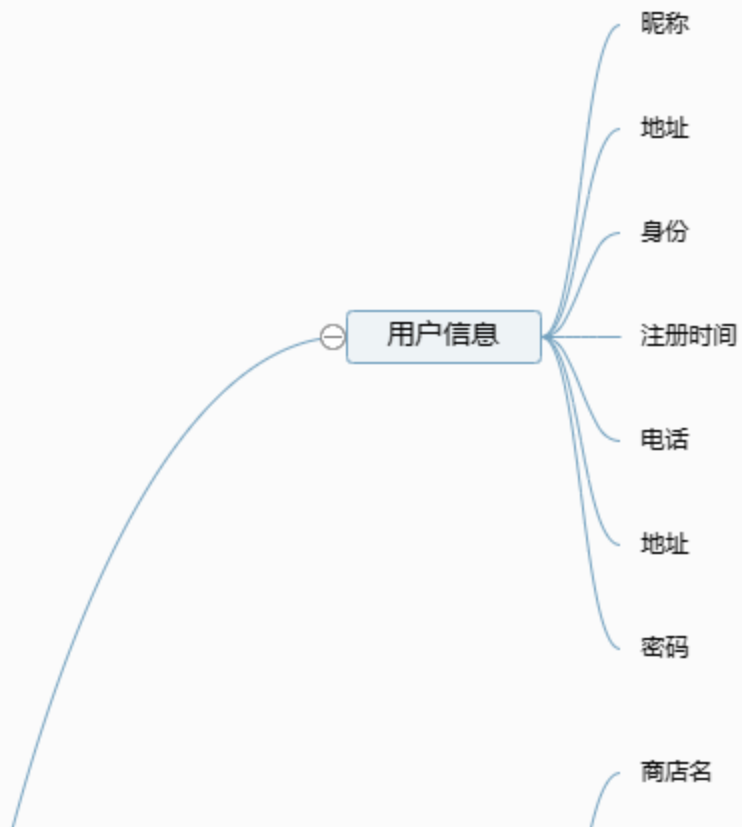
功能结构图
