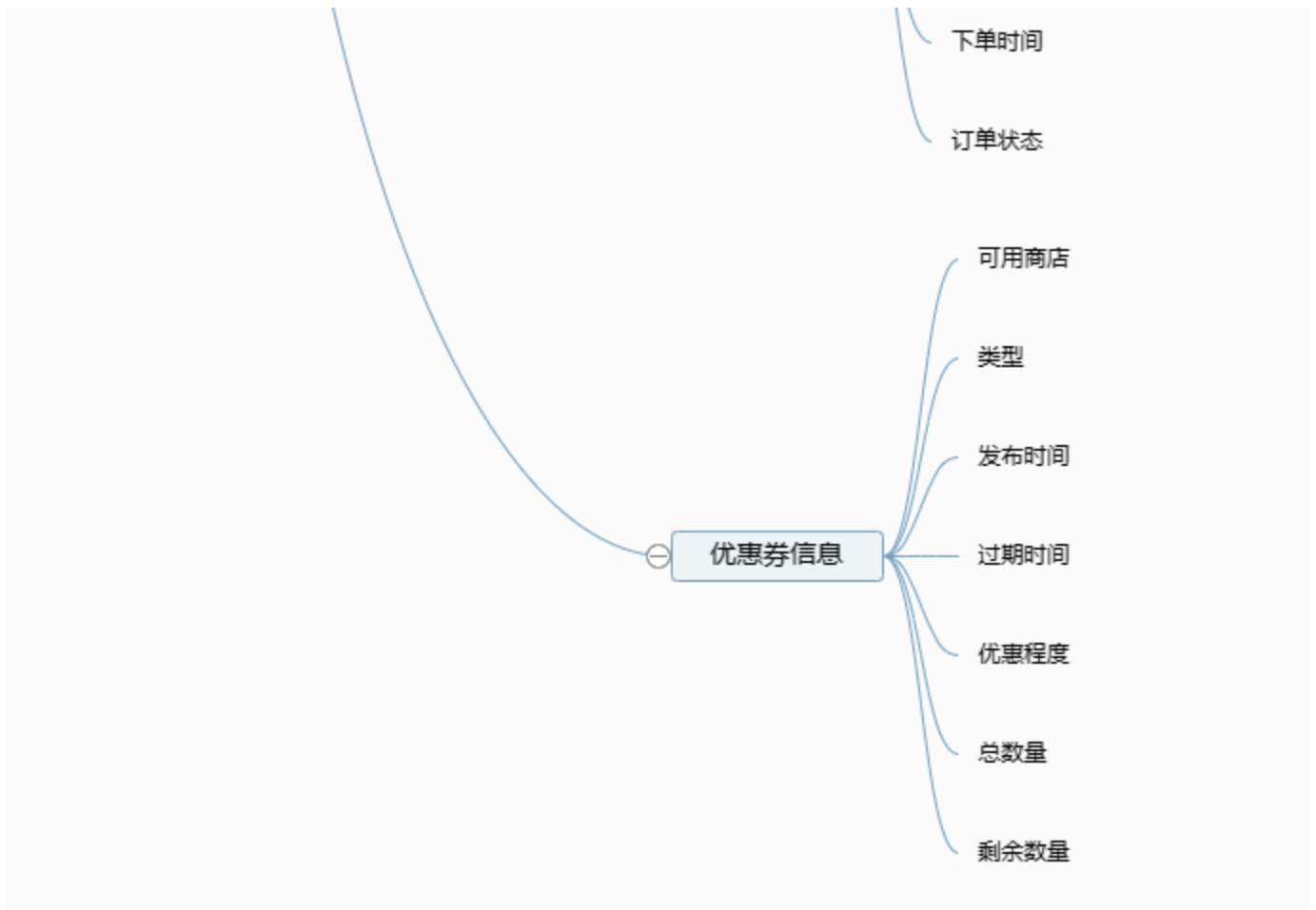
信息结构图
