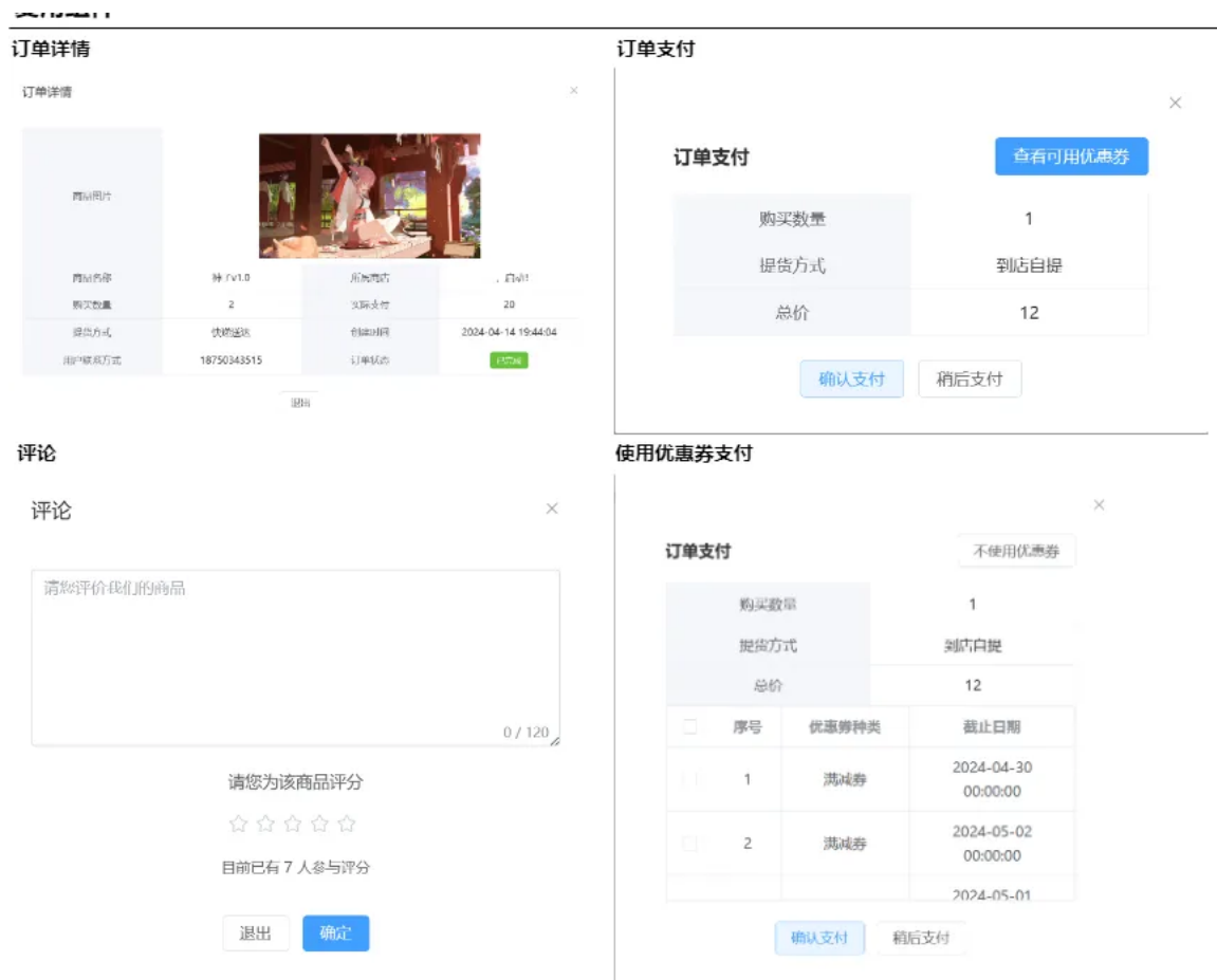
图 4.2.2 复用组件图
