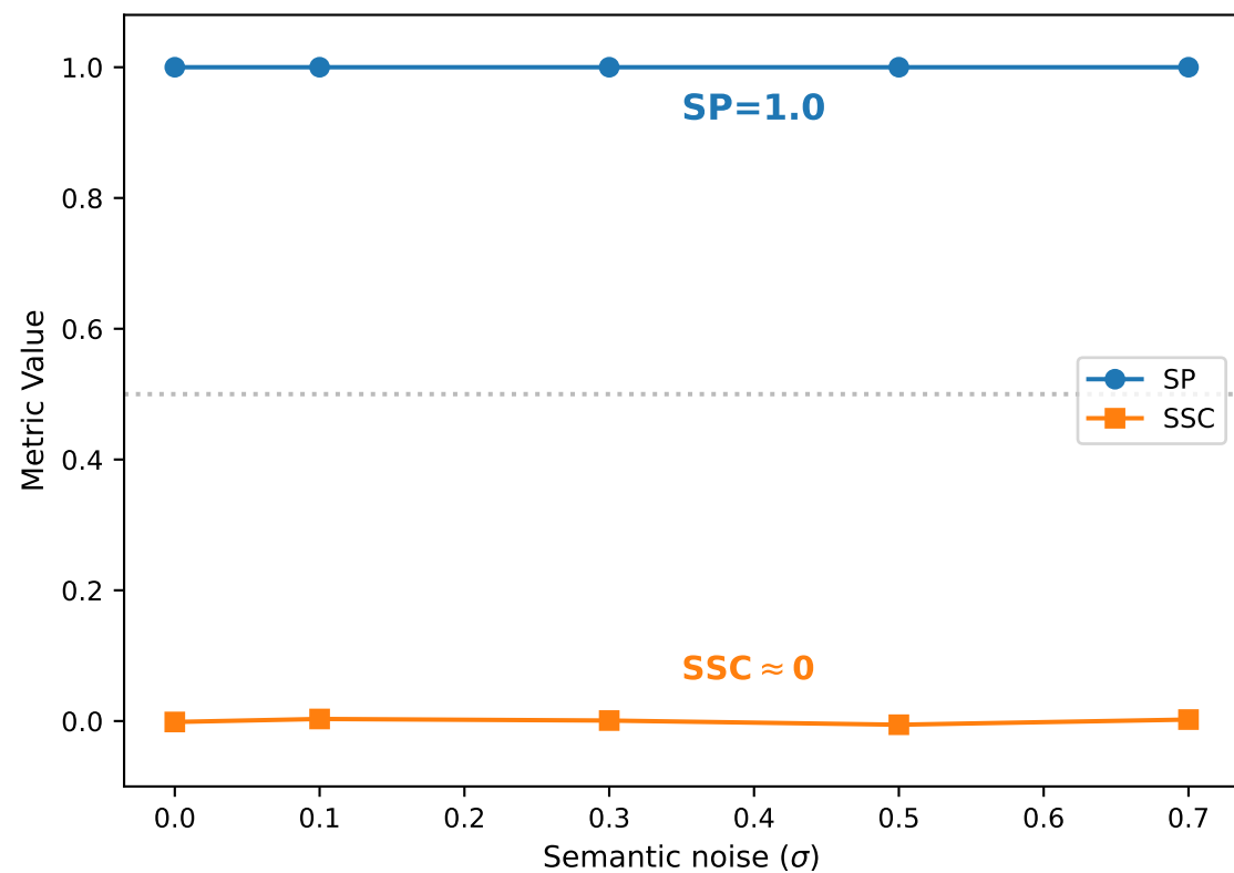
(D) SSC-SP Space: Different axes of variation
