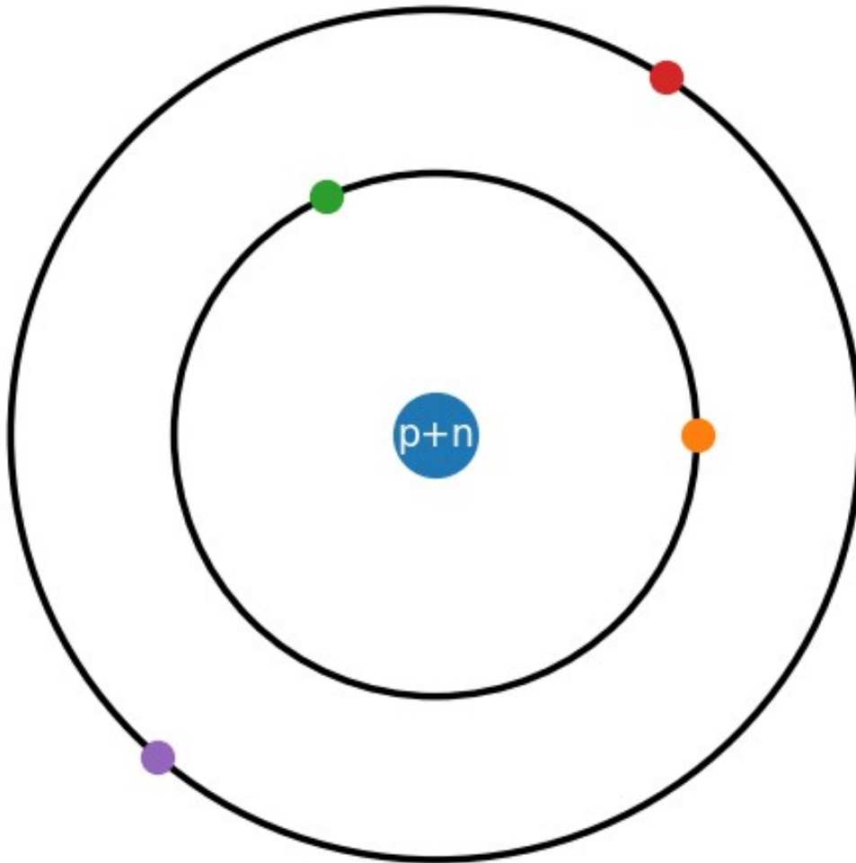
Model atom sederhana: inti dan elektron
