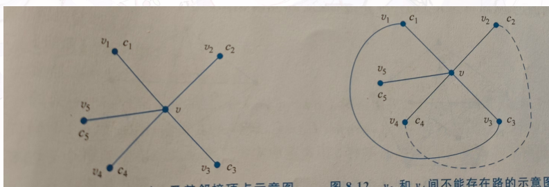
图 8.12 v_1 和 v_3 间不能存在路的示意图
