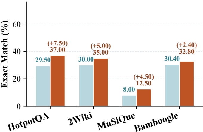
GPT-4o-mini
