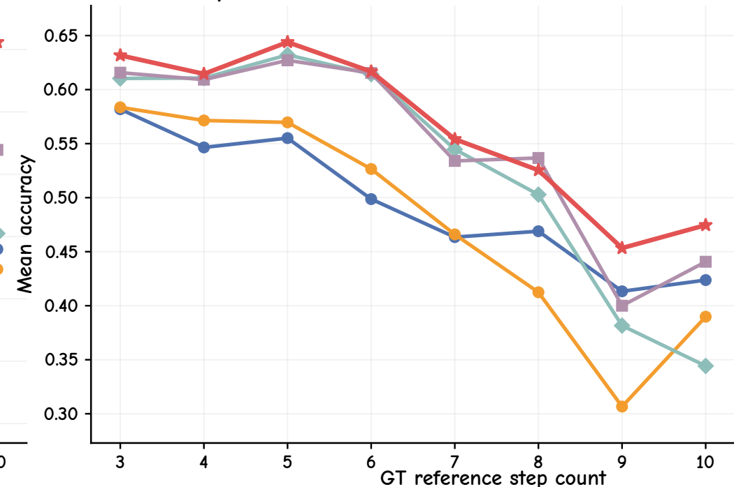
F. Accuracy
