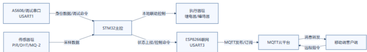
图 3.16 串口与外设数据流向图
