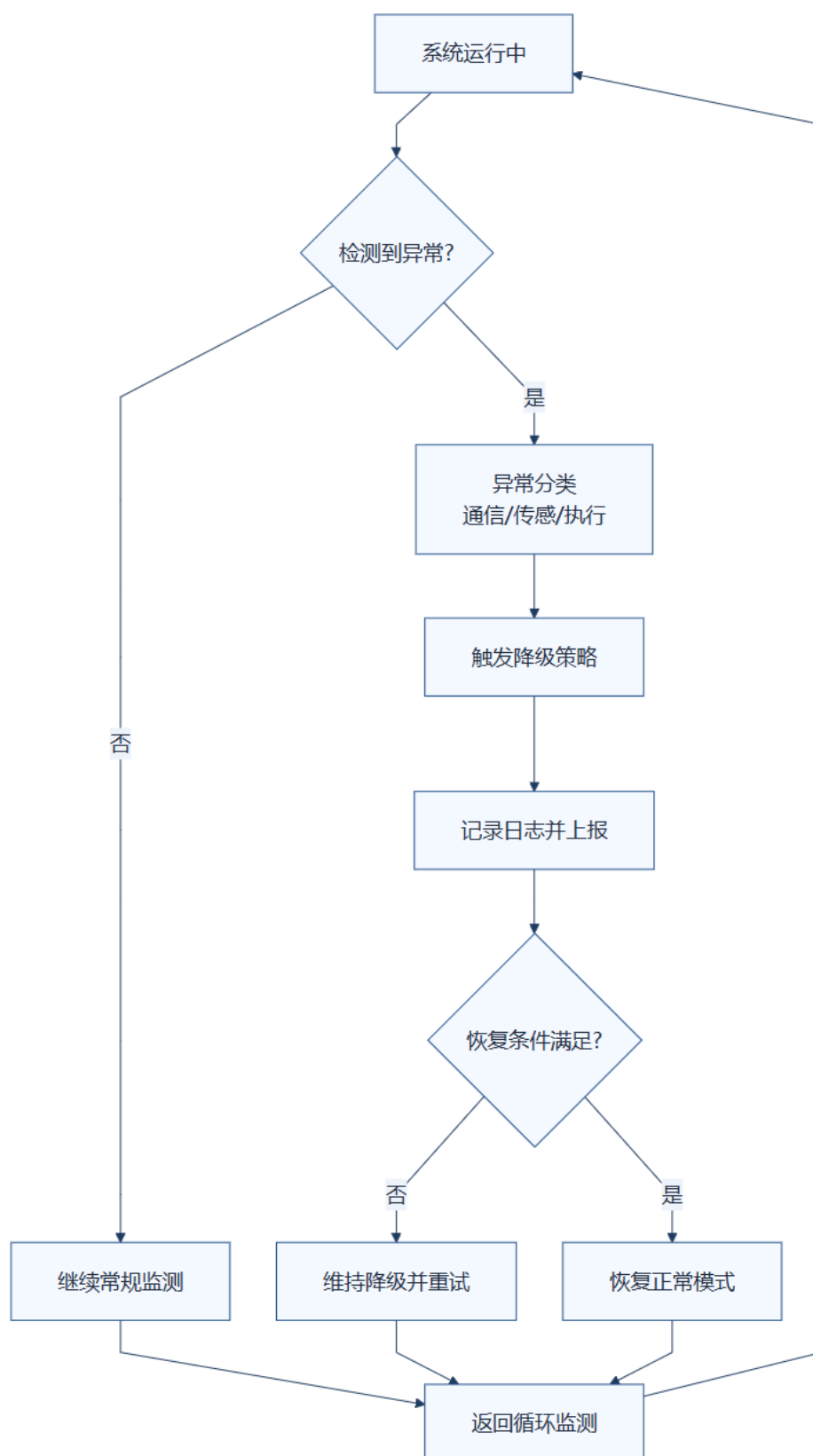
图 4.6 异常处理与恢复流程图
