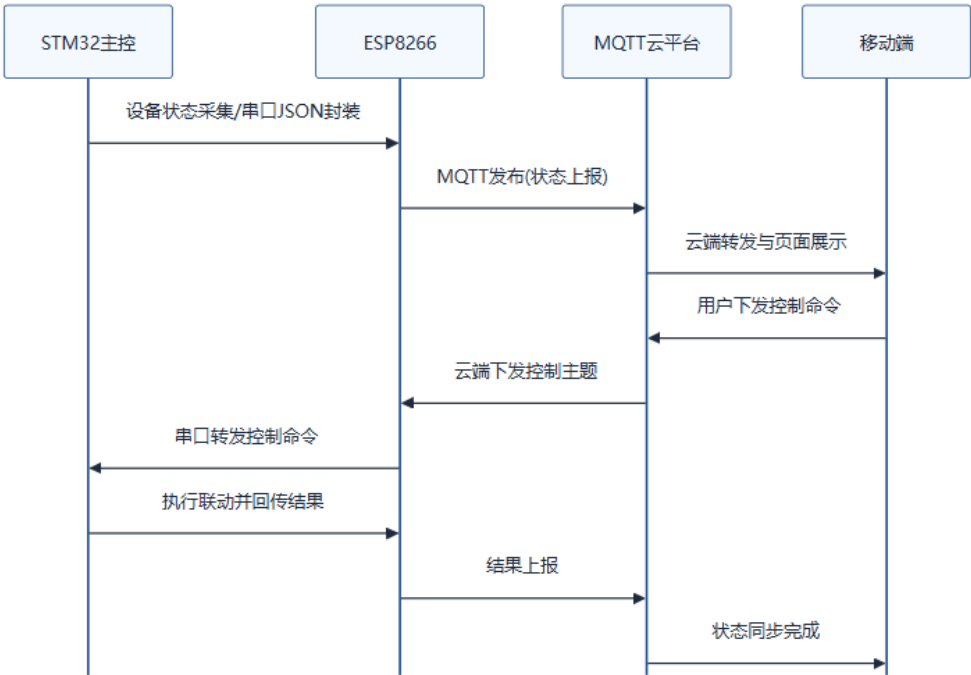
图 4.4 设备与云端通信时序
