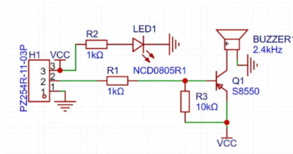
图 3.14 蜂鸣器驱动原理图（原理图）
