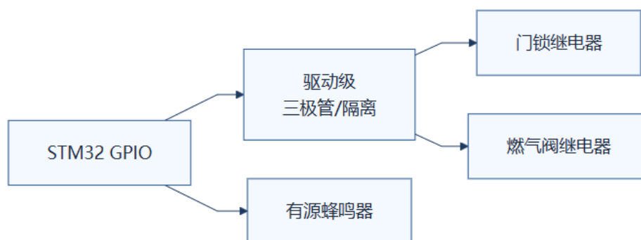
图 3.12 执行器驱动电路示意
