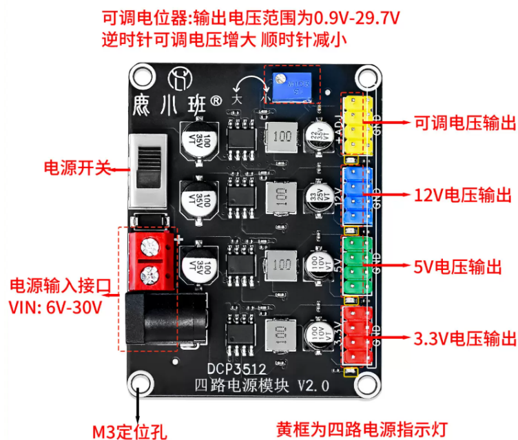
图 3.21 电源模块实物图 (实物图)
