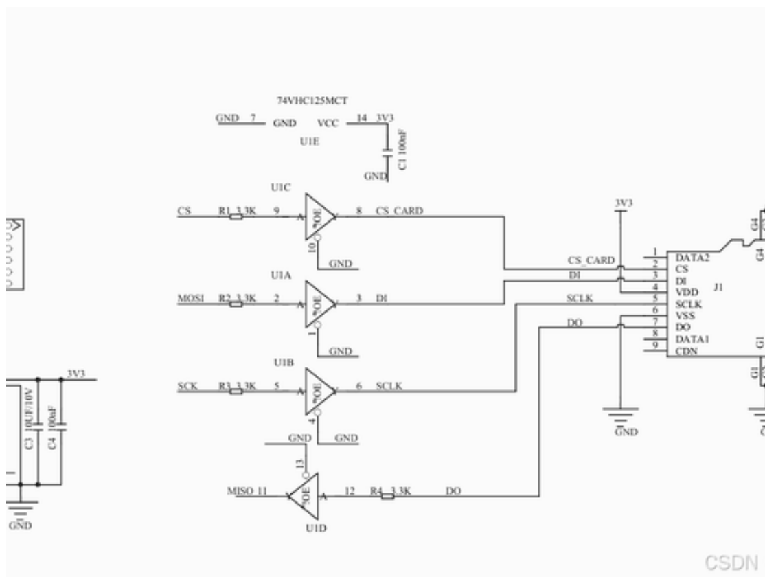
图 3.20 MicroSD 读写模块原理图 (原理图)
