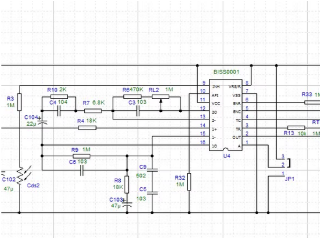
图 3.8 HC-SR501 人体红外模块原理图（原理图）
