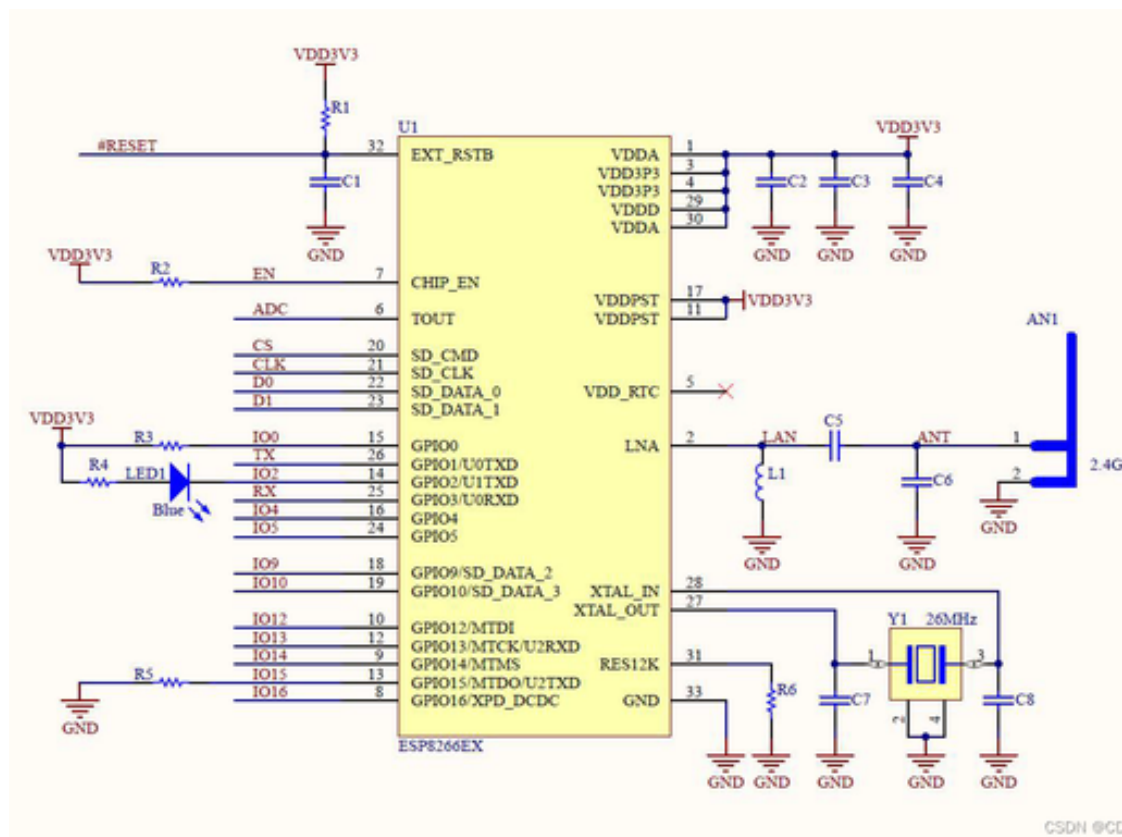
图 3.18 ESP-01S（ESP8266）模块原理图（原理图）
