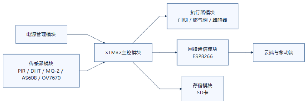
图 3.1 硬件总体连接框图
