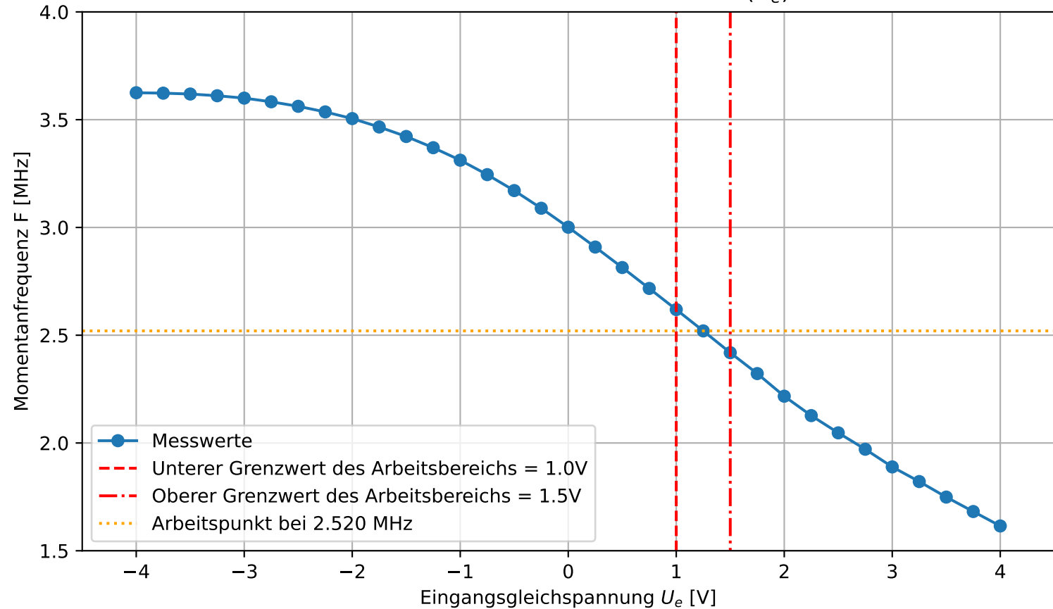
Statische Modulationskennlinie F = f(U_e)
