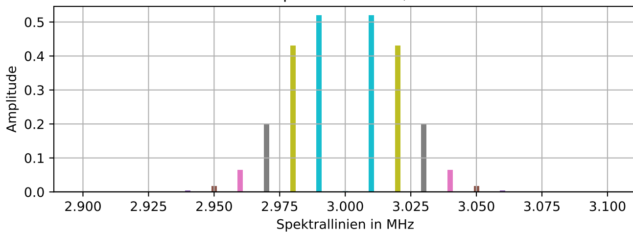
Spektrum m = 2,4
