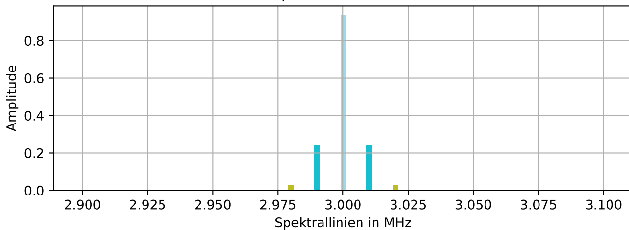
Spektrum m = 0,5
