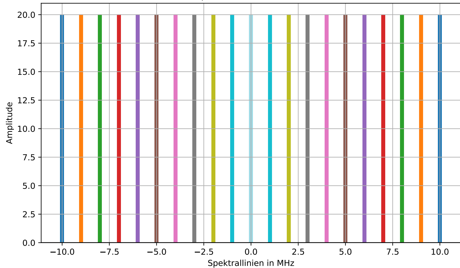
Messspektrum Rechteck m = 10
