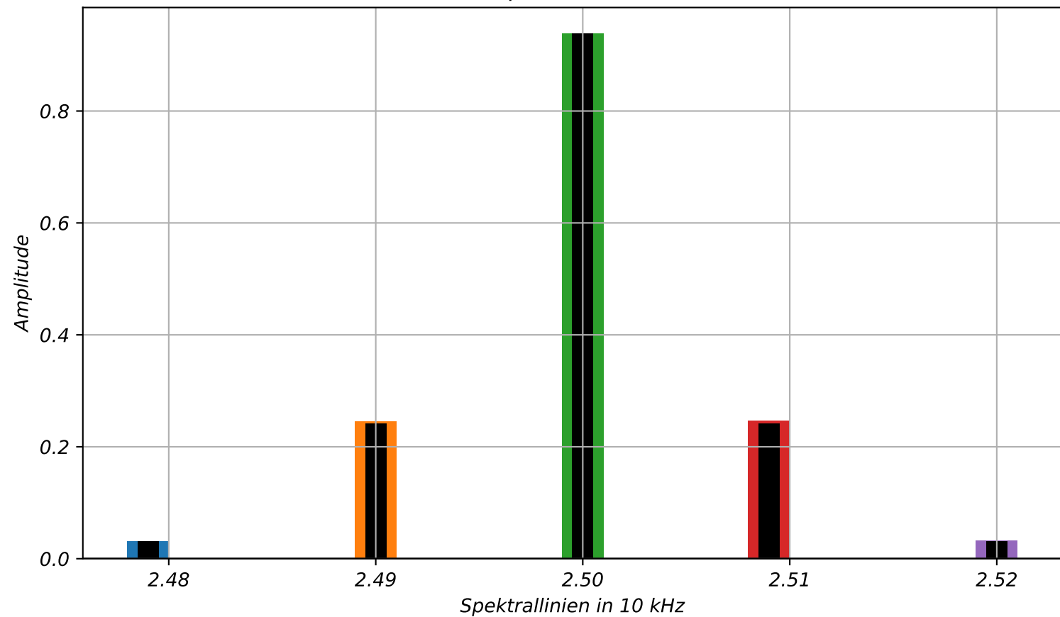
Messspektrum m = 0,5
