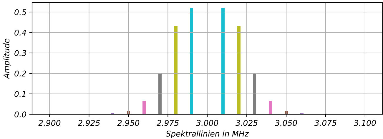
Spektrum m = 2,4
