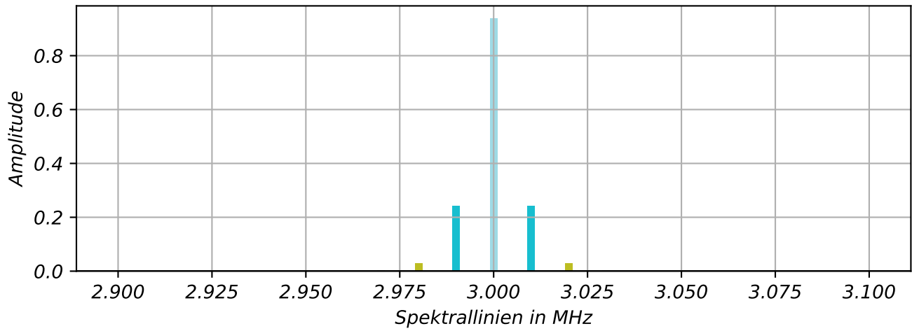
Spektrum m = 0,5
