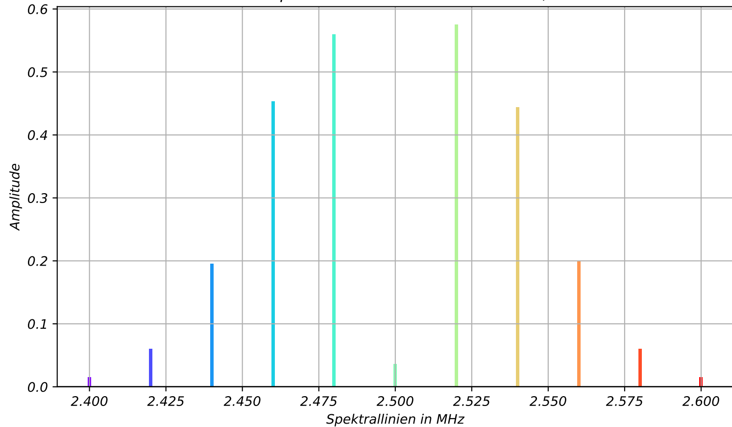
Messspektrum Phasenmodulator m = 2,4
