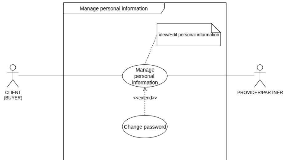
Hình 20: Sơ đồ Use-case Quản lý thông tin cá nhân
