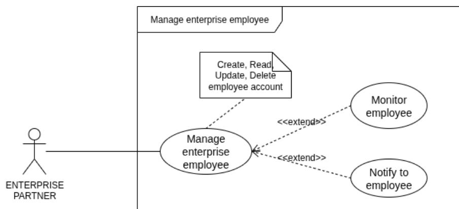
Hình 29: Sơ đồ Use-case Quản lý nhân viên
