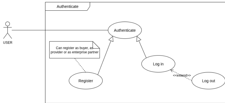
Hình 12: Sơ đồ Use-case xác thực tài khoản
