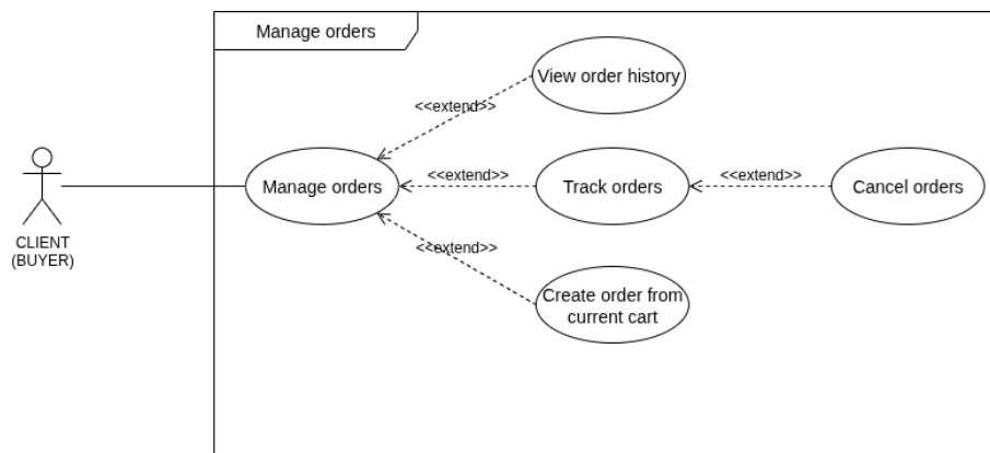
Hình 18: Sơ đồ Use-case Quản lý đơn hàng
