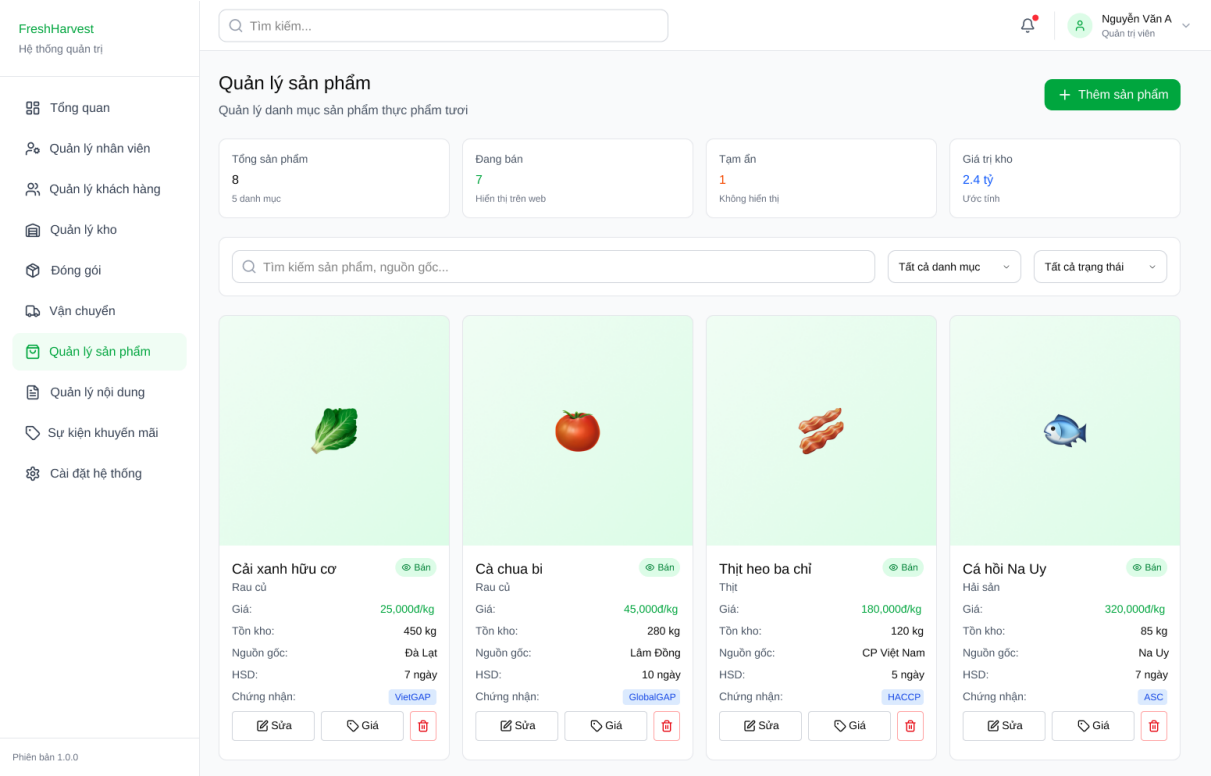
Hình 76: Màn hình quản lý sản phẩm
