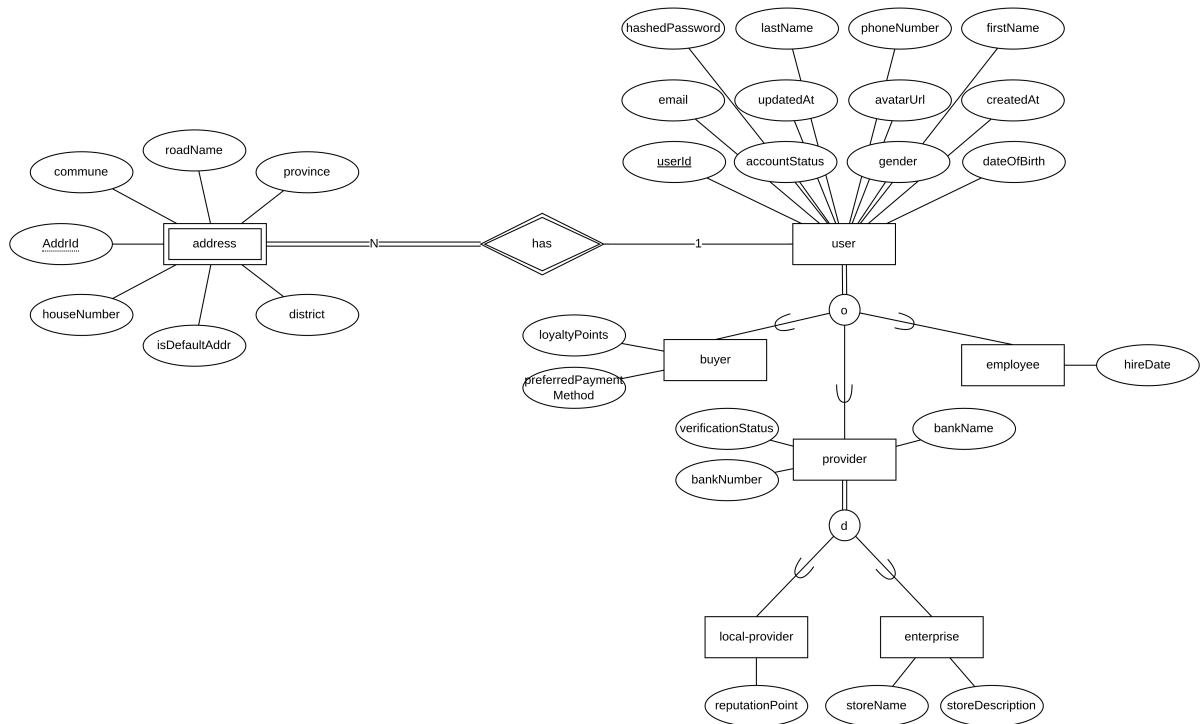
Hình 45: Các thực thể liên quan đến phân loại người dùng
