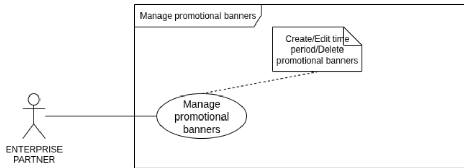
Hình 28: Sơ đồ Use-case Quản lý banner quảng cáo và khuyến mại
