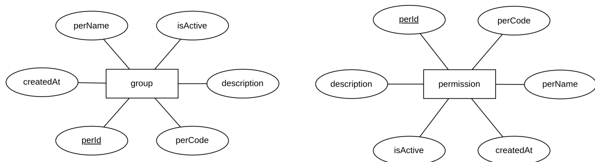
Hình 53: Thực thể liên quan về phân nhóm và quyền cho người dùng
