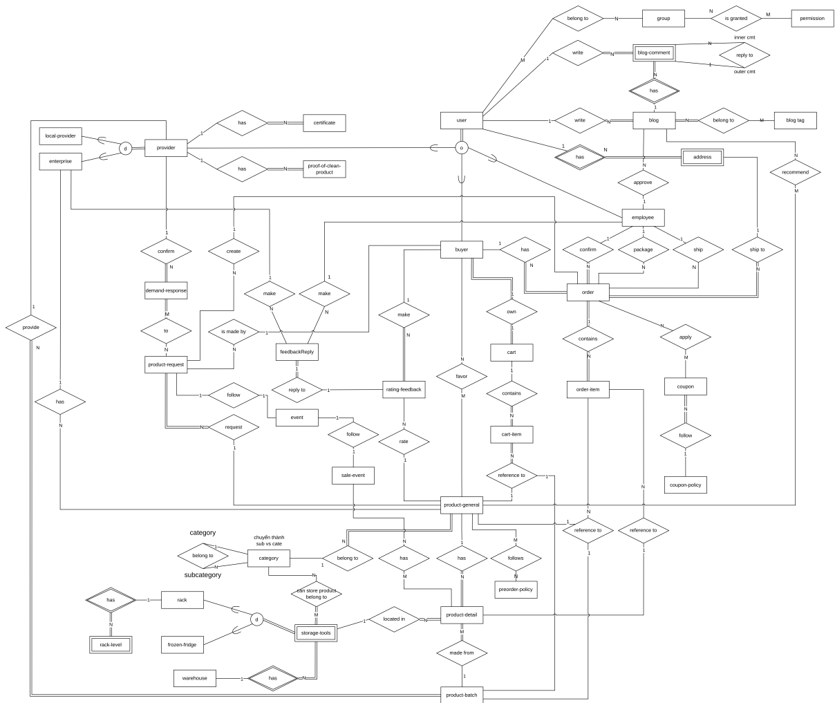
Hình 44: Lược đồ thực thể - mối quan hệ của hệ thống
