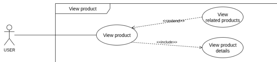
Hình 13: Sơ đồ Use-case Xem sản phẩm
