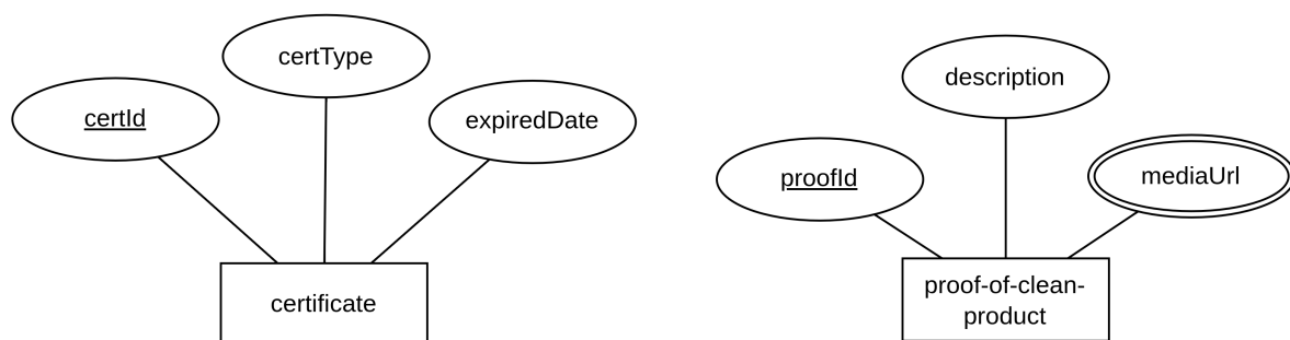
Hình 52: Thực thể liên quan về minh chứng sản phẩm sạch
