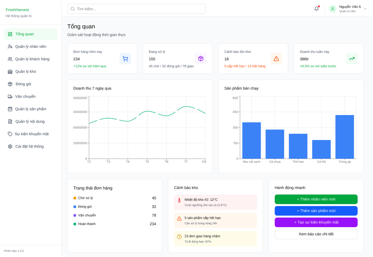
Hình 70: Màn hình dashboard cho nhân viên của cửa hàng
