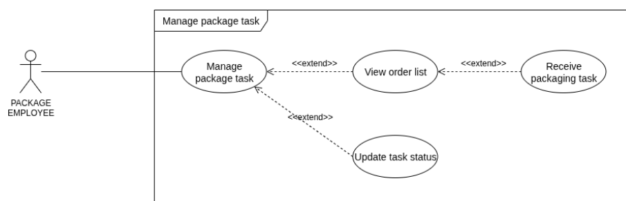
Hình 40: Sơ đồ Use-case Quản lý nhiệm vụ gói hàng
