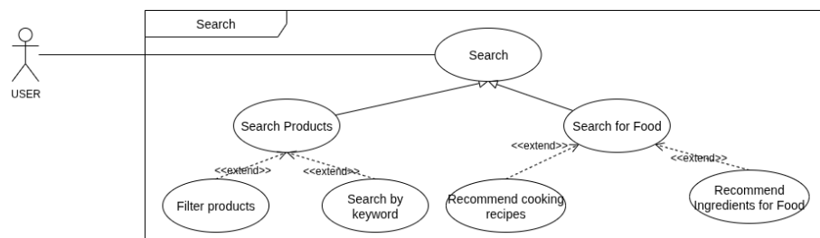
Hình 15: Sơ đồ Use-case Tìm kiếm
