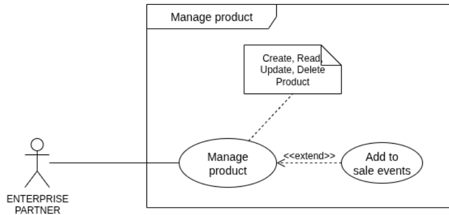
Hình 27: Sơ đồ Use-case Quản lý sản phẩm
