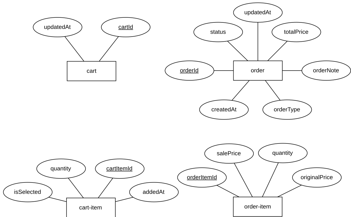
Hình 47: Thực thể liên quan về tác vụ giỏ hàng và đặt hàng
