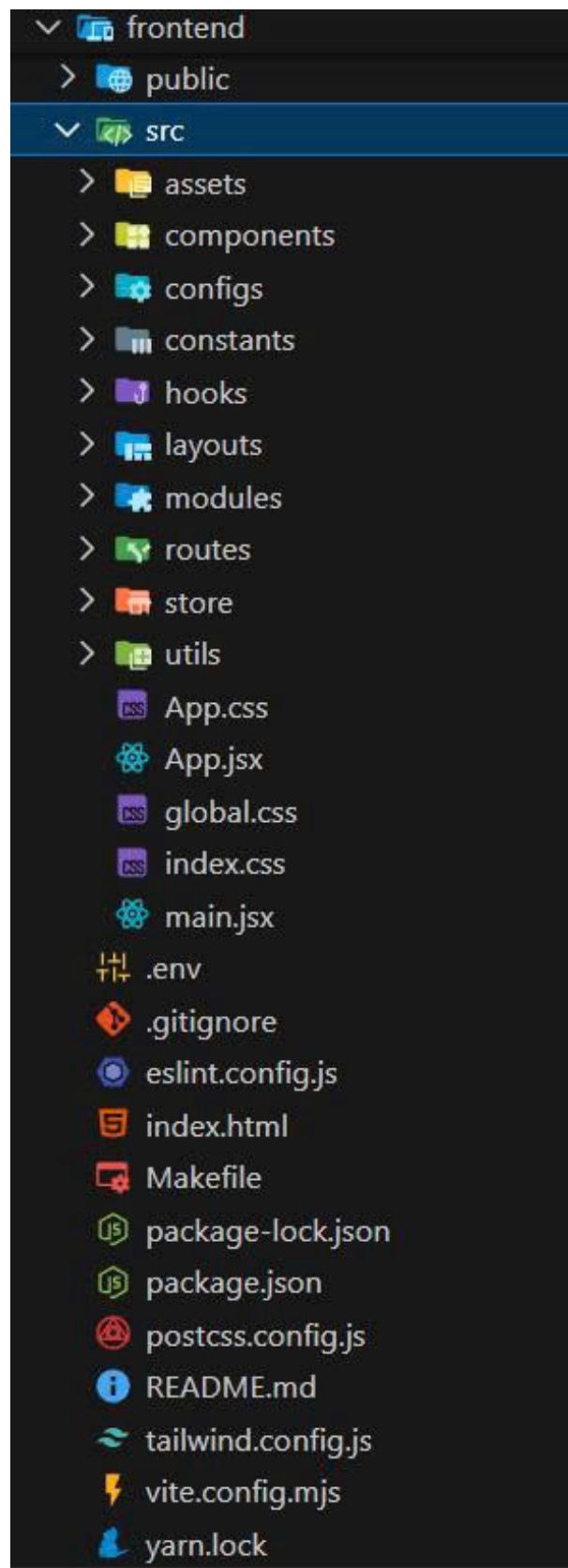
Hình 86: Cấu trúc mã nguồn Front-end
