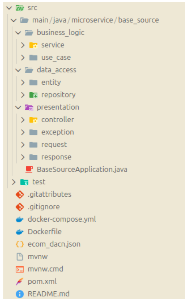
Hình 87: Cấu trúc mã nguồn Back-end
