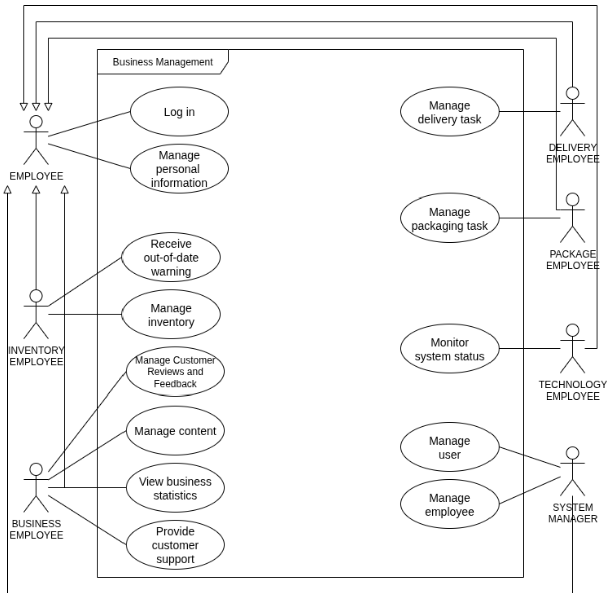
Hình 11: Sơ đồ Use-case tổng quan của hệ thống - phía vận hành kinh doanh
