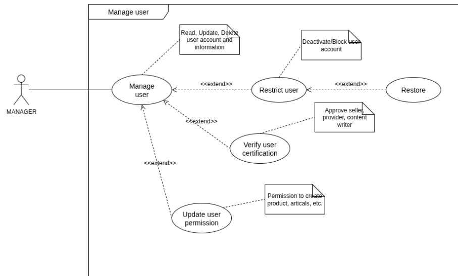
Hình 43: Sơ đồ Use-case Quản lý người dùng
