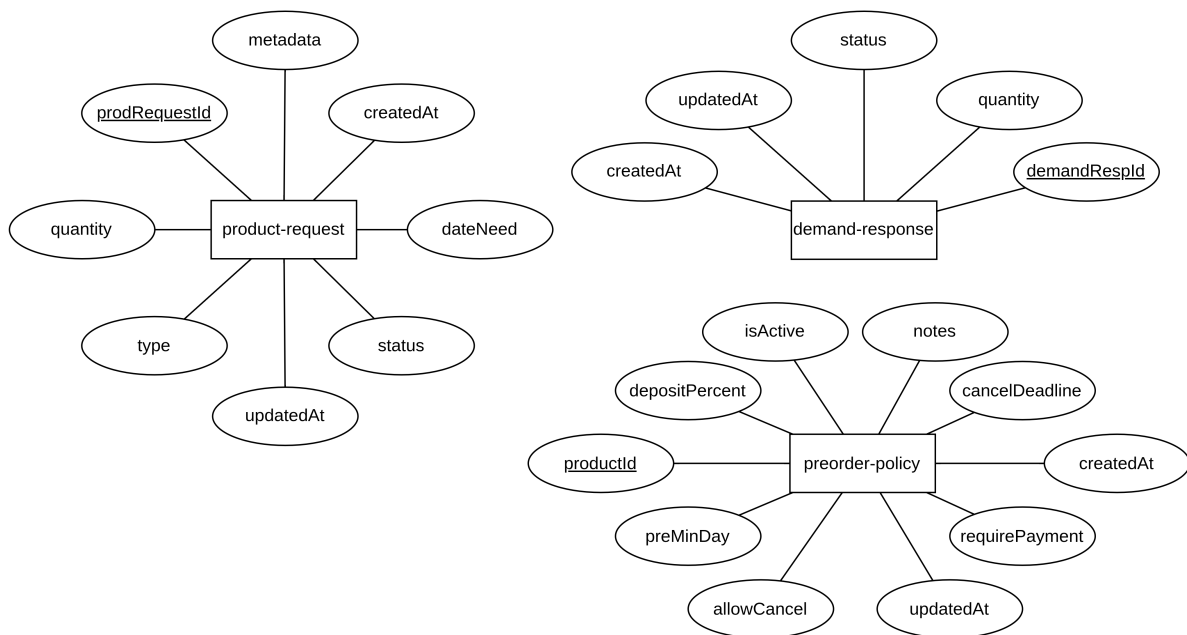
Hình 48: Thực thể liên quan đến tác vụ đặt trước sản phẩm
