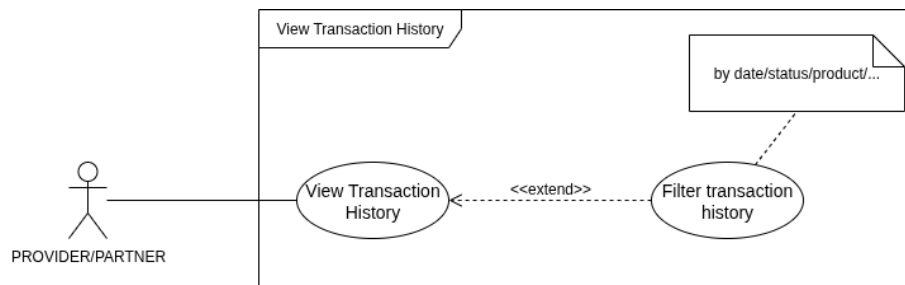
Hình 23: Sơ đồ Use-case Xem lịch sử giao dịch
