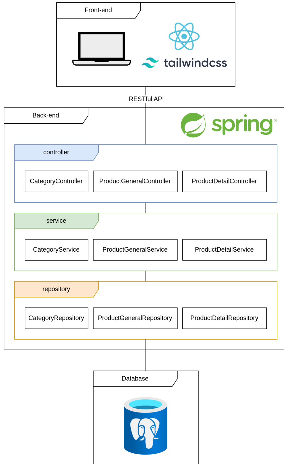
Hình 85: Kiến trúc tổng quan của hệ thống
