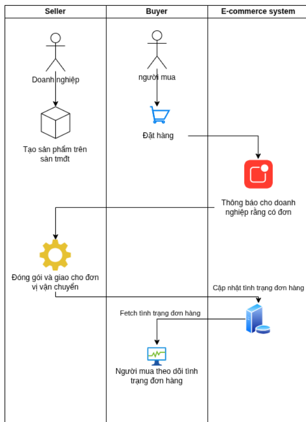
Hình 89: Lưu đồ mua sắm giữa người mua và doanh nghiệp trên sàn TMĐT
