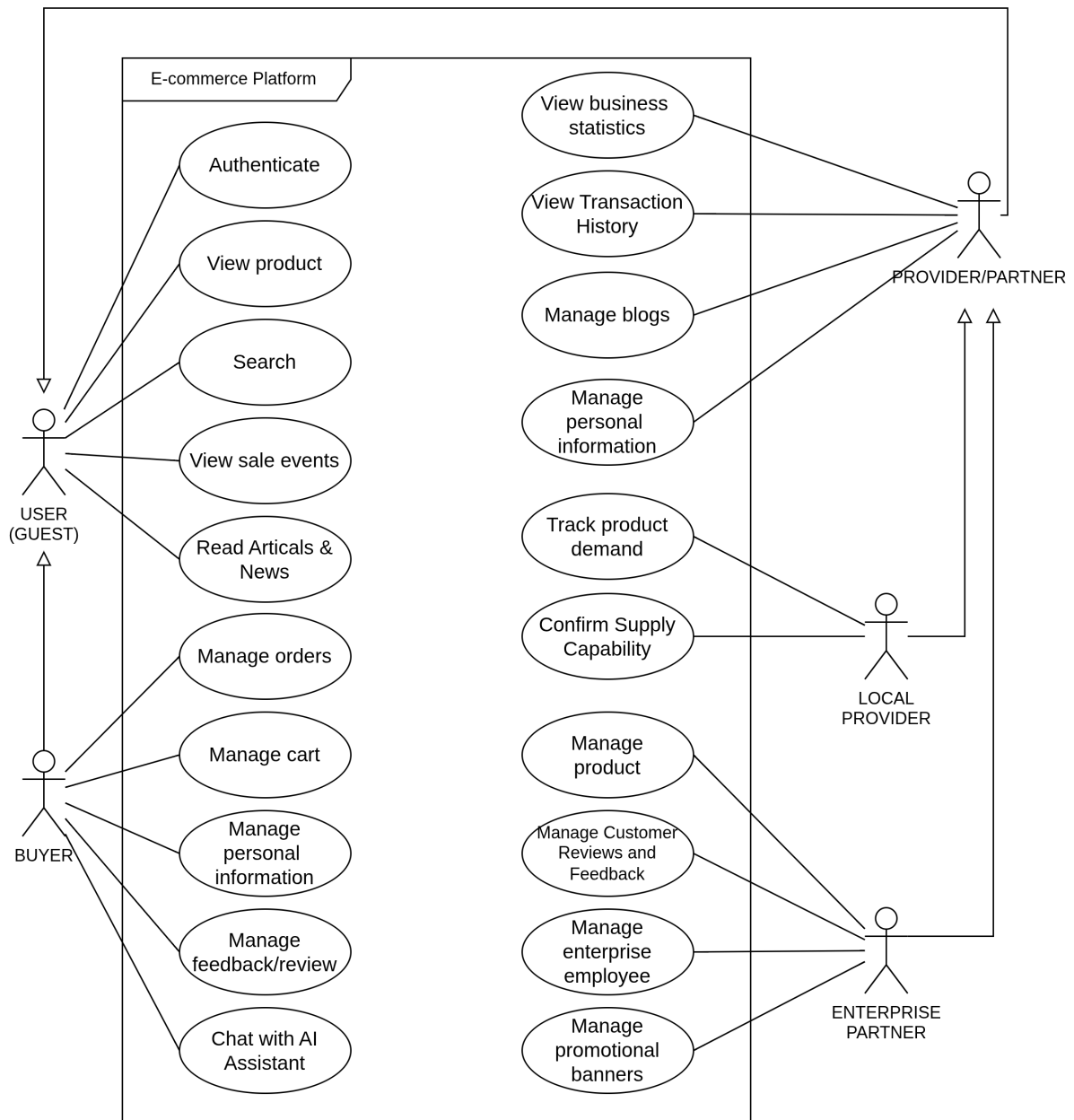
Hình 10: Sơ đồ Use-case tổng quan của hệ thống - phía thương mại điện tử
