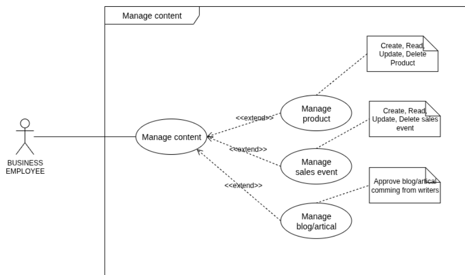
Hình 35: Sơ đồ Use-case Quản lý nội dung
