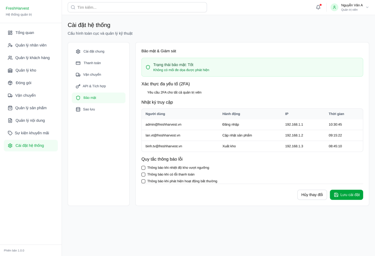
Hình 83: Màn hình cấu hình hệ thống - Cài đặt bảo mật
