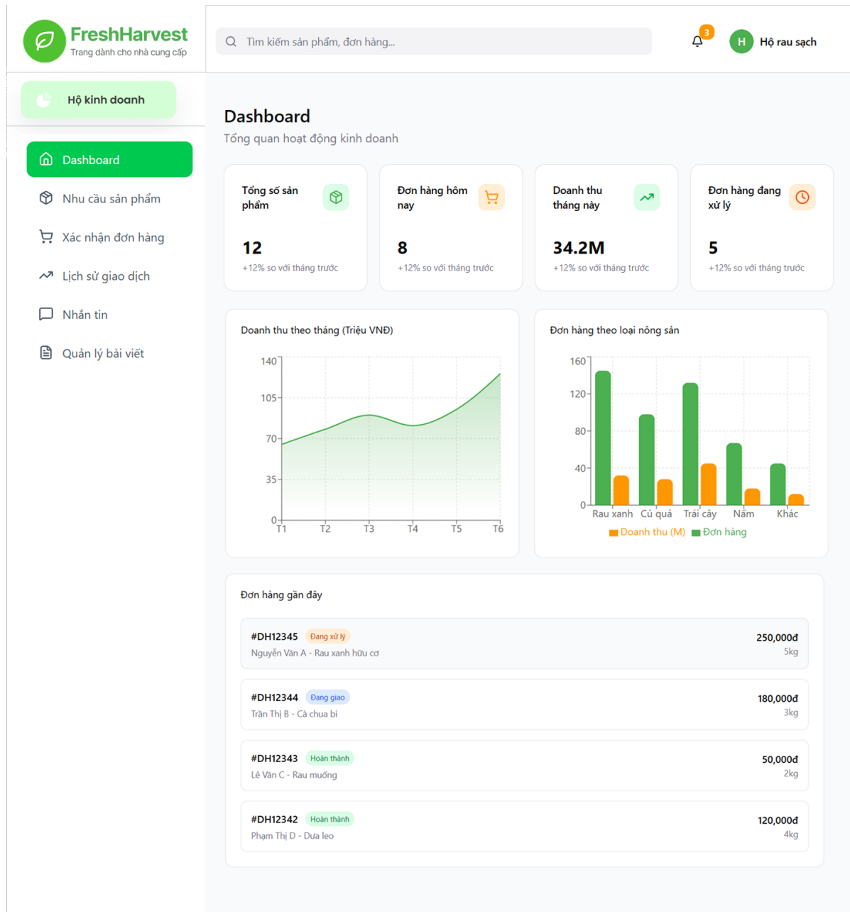
Hình 63: Màn hình dashboard của nhà cung cấp
