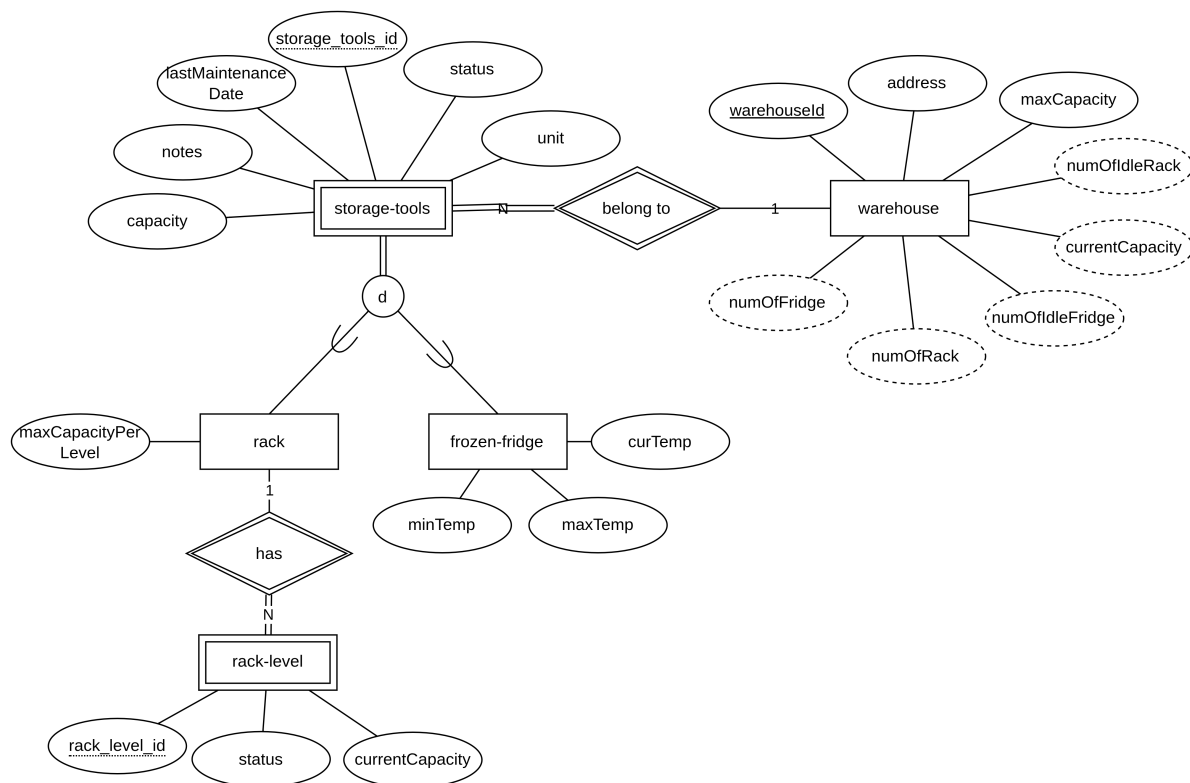
Hình 51: Thực thể liên quan đến nơi lưu trữ sản phẩm
