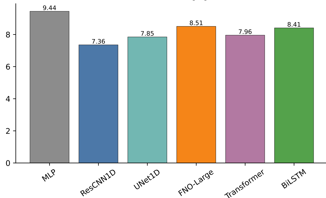
Parameters [M]
