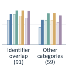
(d) Localization
