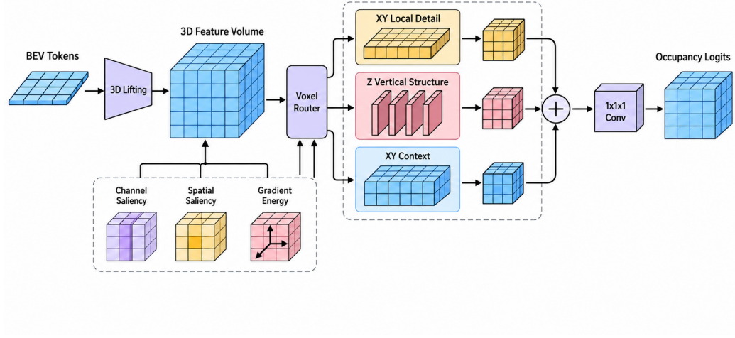
图 6: Agri-AMoE 三维占用解码器。二维 BEV token 经 lifting 形成三维体积，通道/空间显著性和三方向梯度能量共同驱动逐体素路由，三个各向异性专家的输出经残差混合后用于最终分类。
