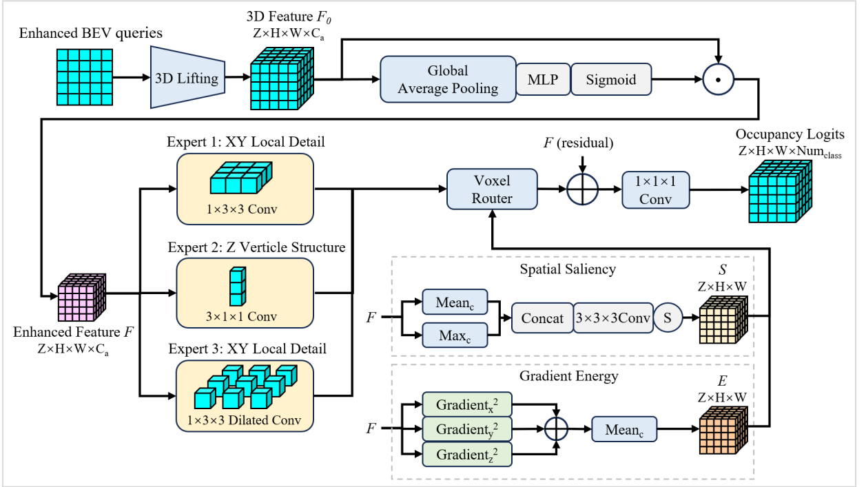
图 7: Agri-AMoE 三维占用解码器。二维 BEV token 经 lifting 形成三维体积, 并首先由通道注意力增强; 增强特征一方面并行输入三个各向异性专家, 另一方面生成空间显著性与三方向梯度能量以计算逐体素路由权重。三个专家输出经加权求和与残差融合后完成最终分类。
