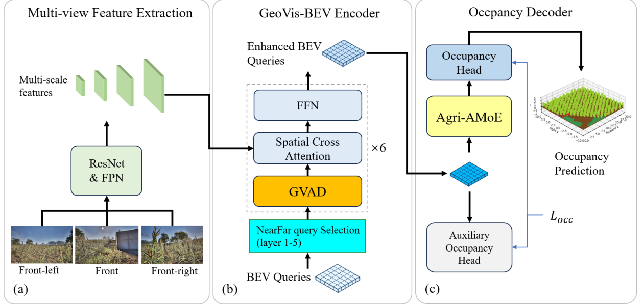
图 4: AgriOcc 总体结构。三路前视图经 ResNet-FPN 提取四尺度特征；六层 GeoVis-BEV 编码器在每层依次执行 GVAD、图像空间交叉注意力与前馈更新，NearFar 在前五层实施近远场查询布局并在第六层前恢复稠密 BEV；三层占用解码器提供多层监督，最后一层通过 Agri-AMoE 将 BEV token 提升为三维特征体，并输出 100 \times 100 \times 25 \times 6 的六类语义 logits。
