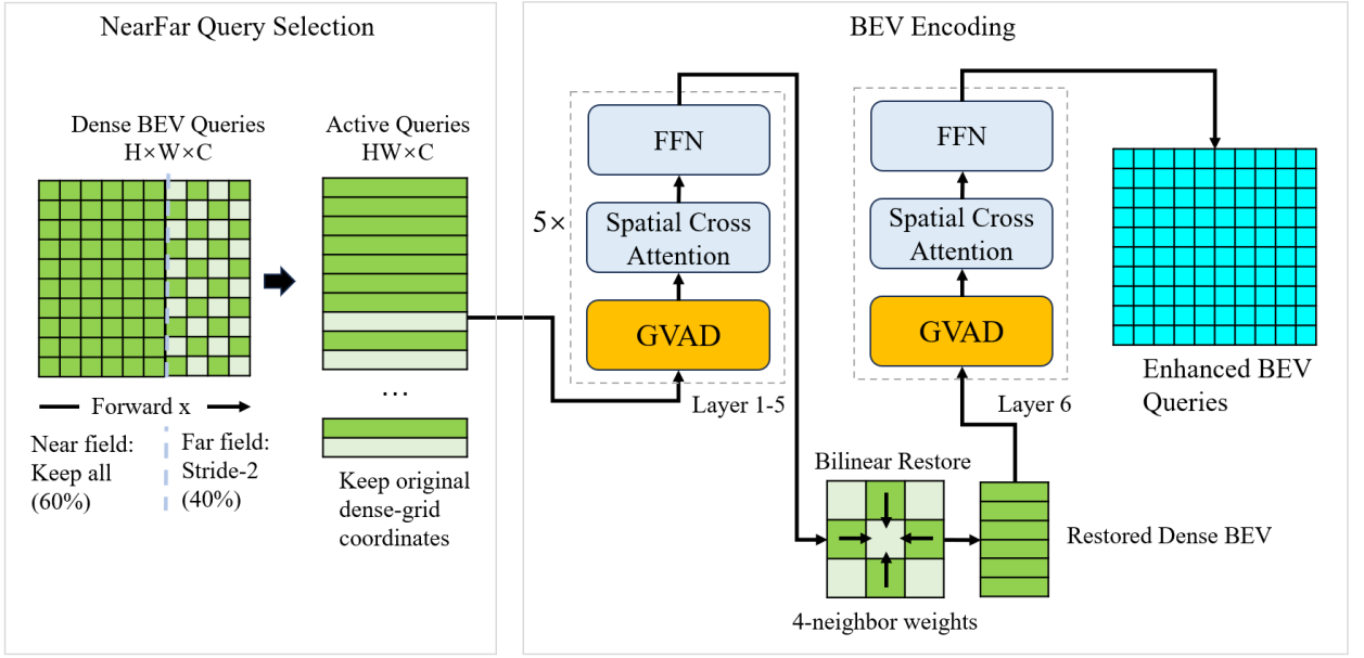
图 5: (a) GeoVis-BEV 编码器整体架构。三路前视图图像经 ResNet-FPN 提取多尺度特征后输入六层编码器；GVAD 在各编码层中更新 BEV token，NearFar 在前五层保留近场稠密查询并对远场规则稀疏采样，恢复为稠密网格后由最后一层完成图像条件细化。
