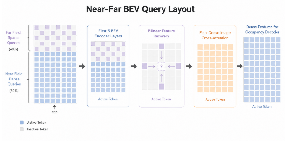
图 4: 近远场 BEV 查询布局。近场保留稠密 token，远场以规则步长稀疏激活；前五个编码层处理 active token，随后通过二维双线性恢复补齐远场，并由最终稠密图像交叉注意力进行特征校正。
