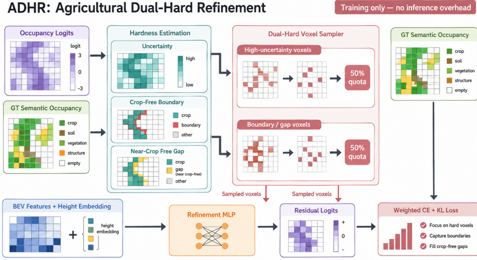
图 3: ADHR 模块。主占用 logits 与 GT 语义共同生成不确定性图、作物-自由空间边界和近作物间隙掩码；双困难采样得到的体素从 BEV 特征读取细化表示，经轻量 MLP 输出辅助残差 logits，并以加权交叉熵和 KL 蒸馏监督训练。
