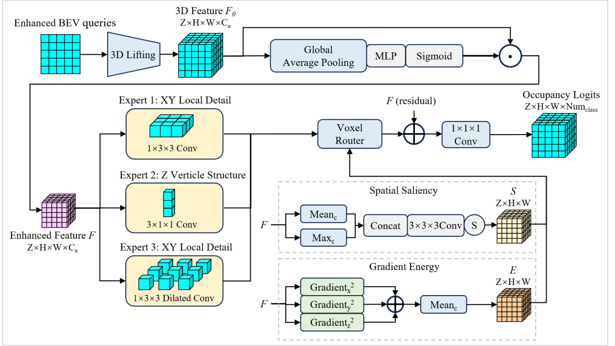
图 7: Agri-AMoE 三维占用解码器。二维 BEV token 经 lifting 形成三维体积, 并首先由通道注意力增强; 增强特征一方面并行输入三个各向异性专家, 另一方面生成空间显著性与三方向梯度能量以计算逐像素路由权重。三个专家输出经加权求和与残差融合后完成最终分类。
