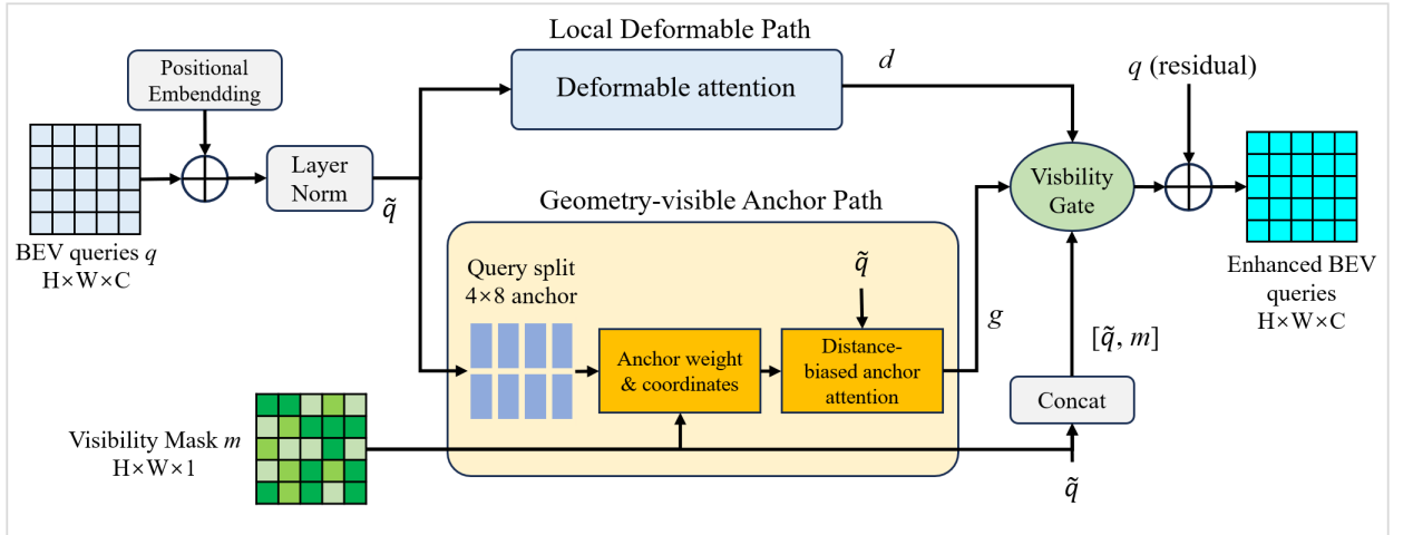
图 6: GVAD 架构。相机投影掩码首先归约为每个 BEV token 的可见性；局部可变形分支根据查询预测采样位置和权重，形成局部 BEV 更新；几何可见锚点分支将 BEV 平面划分为 4 \times 8 个 tile，以特征置信度和可见性加权构建 32 个锚点，并通过距离偏置的多头注意力形成锚点上下文。两条分支经可见性门控和残差连接融合为增强 BEV token。
