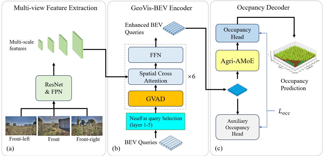
图 4: AgriOcc 总体结构。三路前视图像经 ResNet-FPN 提取四尺度特征；六层 GeoVis-BEV 编码器在每层依次执行 GVAD、图像空间交叉注意力与前馈更新，NearFar 在前五层实施近远场查询布局并在第六层前恢复稠密 BEV；三层占用解码器提供多层监督，最后一层通过 Agri-AMoE 将 BEV token 提升为三维特征体，并输出 100 \times 100 \times 25 \times 6 的六类语义 logits。
