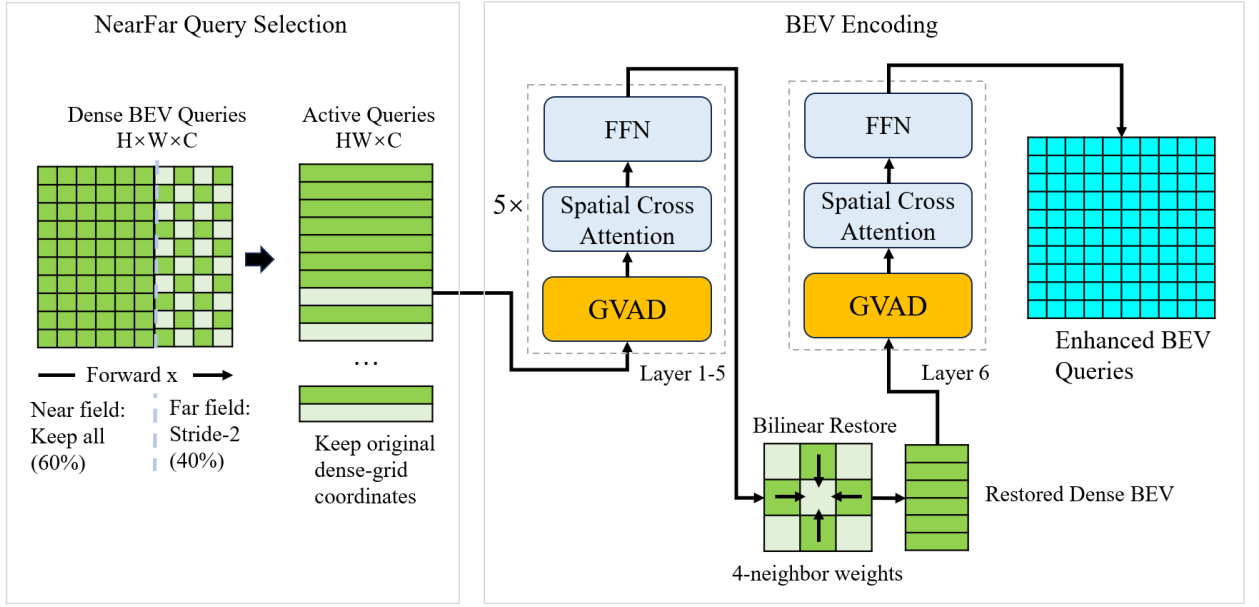
图 5: GeoVis-BEV 编码器整体架构。三路前视图像经 ResNet-FPN 提取多尺度特征后输入六层编码器；GVAD 在各编码层中更新 BEV token，NearFar 在前五层保留近场稠密查询并对远场规则稀疏采样，恢复为稠密网格后由最后一层完成图像条件细化。
