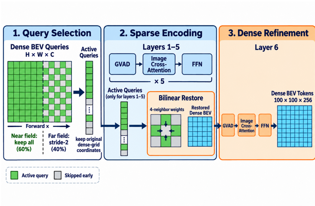
图 7: NearFar 架构。输入稠密 BEV 网格沿前向距离划分为近场与远场，远场按步长 2 下采样激活。所有 active token 保留其原始稠密网格坐标，并在前五层进行稀疏编码；随后，未激活远场位置由相邻四个 active token 的双线性权重恢复为完整网格。
