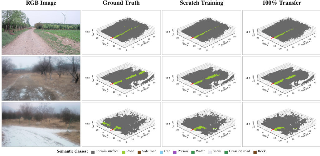
图 10: ORAD-3D 上的定性迁移比较。每行对应同一官方测试样本；从左至右为输入 RGB 图像、真值标签、使用全部 ORAD-3D 训练数据的从头训练结果，以及 AgriOcc-Dataset 预训练后在全部 ORAD-3D 训练数据上迁移的结果（100% Transfer）。
