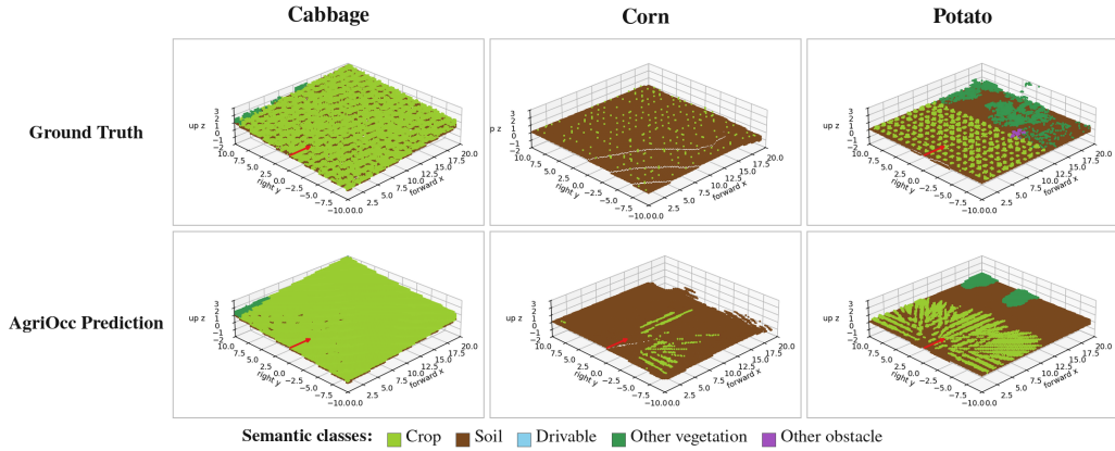
图 11: AgriOcc-Dataset 上的局限性示例。第一行为真值标签，第二行为对应的 AgriOcc 预测；三列从左至右分别为卷心菜、玉米和马铃薯场景。密集作物的株间空隙易被预测为连通区域，而苗期等小尺度作物容易出现漏检或范围不足。
