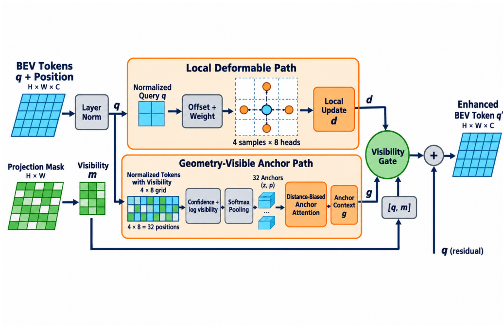
图 6: GVAD 架构。相机投影掩码首先归约为每个 BEV token 的可见性；局部可变形分支根据查询预测采样位置和权重，形成局部 BEV 更新；几何可见锚点分支将 BEV 平面划分为 4 \times 8 个 tile，以特征置信度和可见性加权构建 32 个锚点，并通过距离偏置的多头注意力形成锚点上下文。两条分支经可见性门控和残差连接融合为增强 BEV token。
