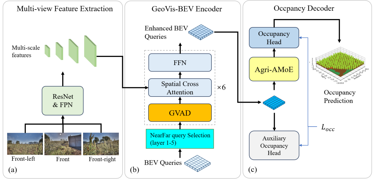
图 4: AgriOcc 总体结构。三路前视图图像经 ResNet-FPN 提取四尺度特征；六层 GeoVis-BEV 编码器在每层依次执行 GVAD、图像空间交叉注意力与前馈更新，NearFar 在前五层实施近远场查询布局并在第六层前恢复稠密 BEV；三层占用解码器提供多层监督，最后一层通过 Agri-AMoE 将 BEV token 提升为三维特征体，并输出 100 \times 100 \times 25 \times 6 的六类语义 logits。
