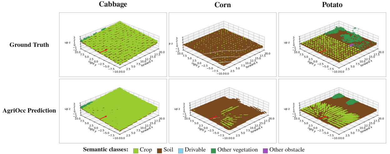
图 10: AgriOcc-Dataset 上的局限性示例。第一行为真值标签，第二行为对应的 AgriOcc 预测；三列从左至右分别为卷心菜、玉米和马铃薯场景。密集作物的株间间隙易被预测为连通区域，而苗期等小尺度作物容易出现漏检或范围不足。
