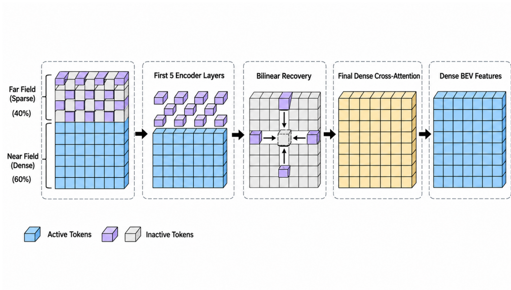
图 4: 近远场 BEV 查询布局。近场保留稠密 token，远场以规则步长稀疏激活；前五个编码层处理 active token，随后通过二维双线性恢复补齐远场，并由最终稠密图像交叉注意力进行特征校正。
