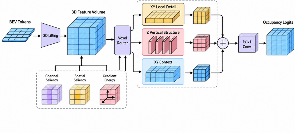
图 3: Agri-AMoE 三维占用解码器。最终 BEV token 被提升为三维特征体；通道显著性、空间显著性与 x/y/z 方向梯度能量输入逐体素路由器，分别激活平面局部细节、垂直结构和大范围平面上下文专家。三个专家的加权结果经残差混合与 1 \times 1 \times 1 分类卷积产生语义体素 logits。
