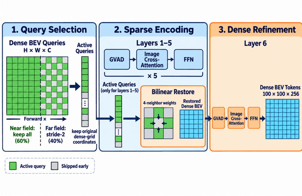
图 5: NearFar 架构。输入稠密 BEV 网格沿前向距离划分为近场与远场，远场按步长 2 下采样激活。所有 active token 保留其原始稠密网格坐标，并在前五层进行稀疏编码；随后，未激活远场位置由相邻四个 active token 的双线性权重恢复为完整网格。
