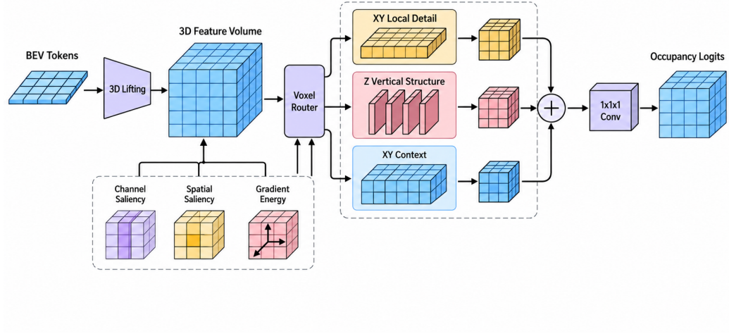
图 6: Agri-AMoE 三维占用解码器。最终 BEV token 被提升为三维特征体；通道显著性、空间显著性与 x/y/z 方向梯度能量输入逐体素路由器，分别激活平面局部细节、垂直结构和大范围平面上下文专家。三个专家的加权结果经残差混合与 1 \times 1 \times 1 分类卷积产生语义体素 logits。
