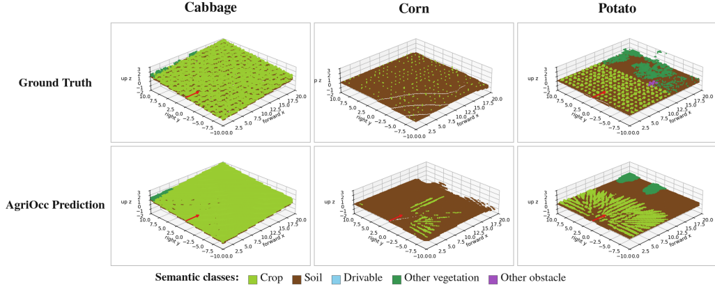
图 10: AgriOcc-Dataset 上的局限性示例。第一行为真值标签，第二行为对应的 AgriOcc 预测；三列从左至右分别为卷心菜、玉米和马铃薯场景。密集作物的株间间隙易被预测为连通区域，而苗期等小尺度作物容易出现漏检或范围不足。
