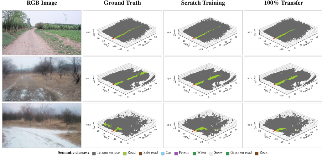
图 9: ORAD-3D 上的定性迁移比较。每行对应同一官方测试样本；从左至右为输入 RGB 图像、真值标签、使用全部 ORAD-3D 训练数据的从头训练结果，以及 AgriOcc-Dataset 预训练后在全部 ORAD-3D 训练数据上迁移的结果（100% Transfer）。
