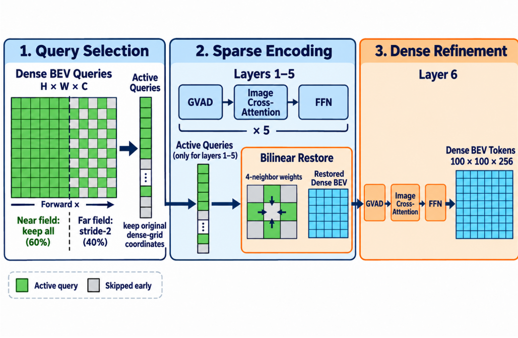
图 6: NearFar 架构。输入稠密 BEV 网格沿前向距离划分为近场与远场，远场按步长 2 下采样激活。所有 active token 保留其原始稠密网格坐标，并在前五层进行稀疏编码；随后，未激活远场位置由相邻四个 active token 的双线性权重恢复为完整网格。
